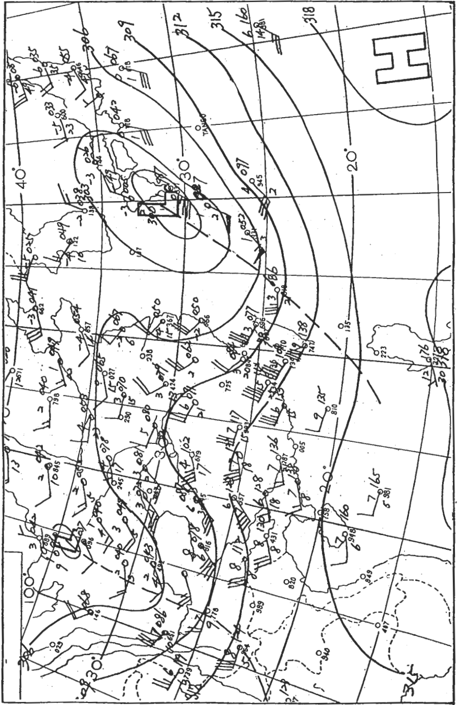
圖九：使我國華中低層弱風區消失導致南支噴射氣流遂雜造成台灣良好之天氣圖 70年3月2日 0000Z 700mb 圖
