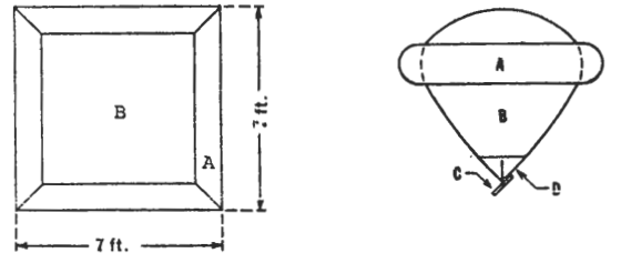
圖 3 火箭氣球傘
