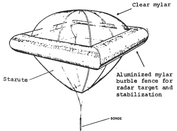
圖 4 火箭穩定傘
