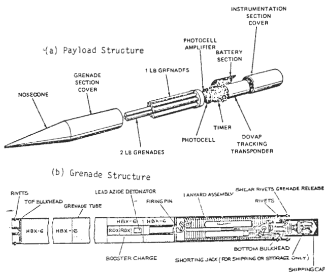
圖8. 聲波彈之構造
