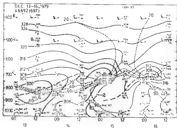
圖 10. 1979 年 12 月 13 - 16 日 (A) 石垣島 (B) 台北及桃園之相當位溫 (實線, °K) 與相對濕度 (虛線, %) 時間剖面圖。粗虛線表潛在不穩定層頂。
