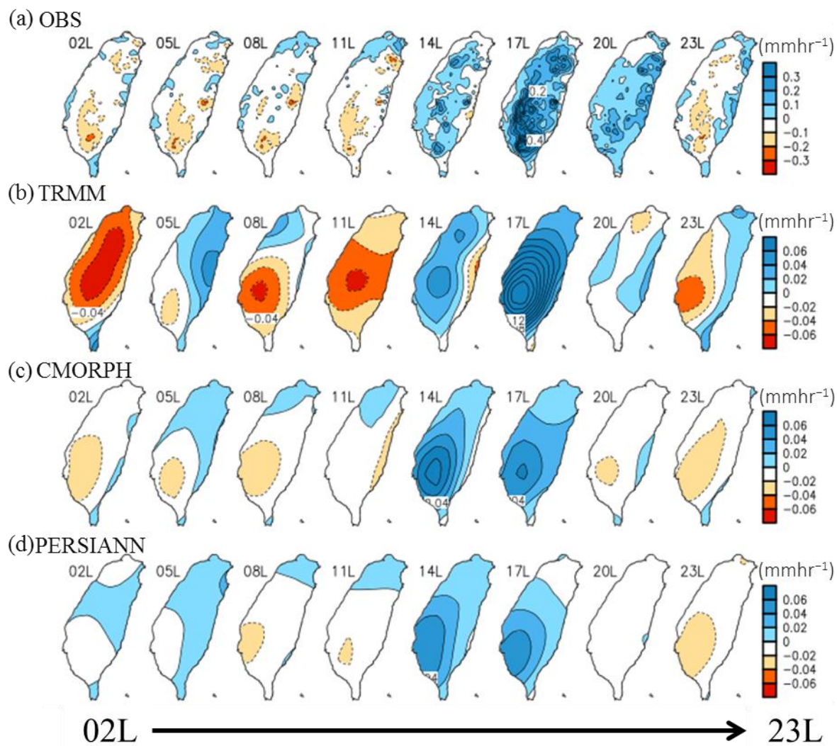
圖 4 類似圖 2，但為秋季降雨日變化量之時間、空間變化。單位為 mm hr -1 。
