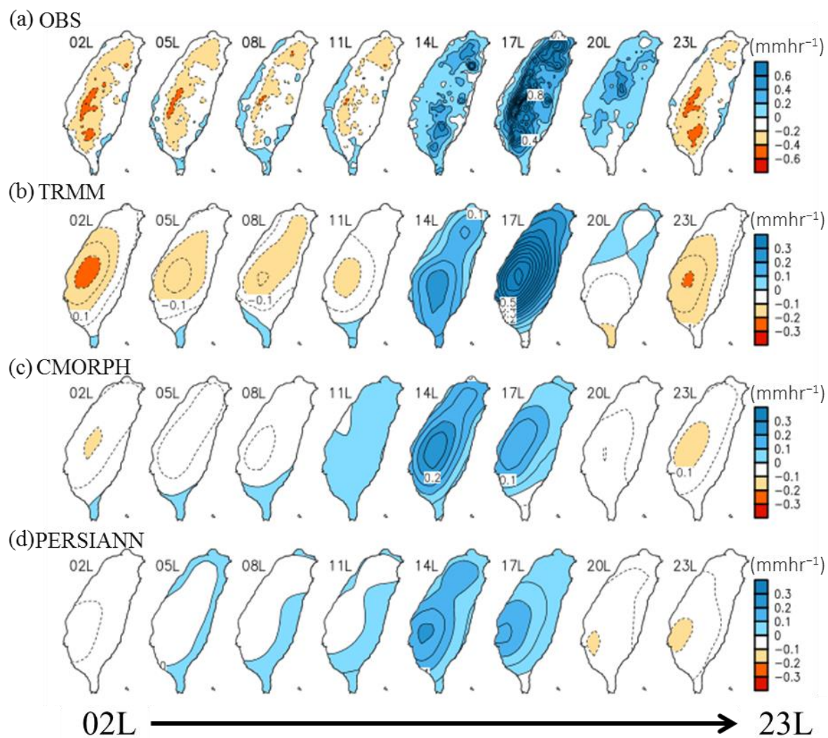
圖 3 類似圖 2，但為夏季降雨日變化量之時間、空間變化。單位為 mm hr -1 。
