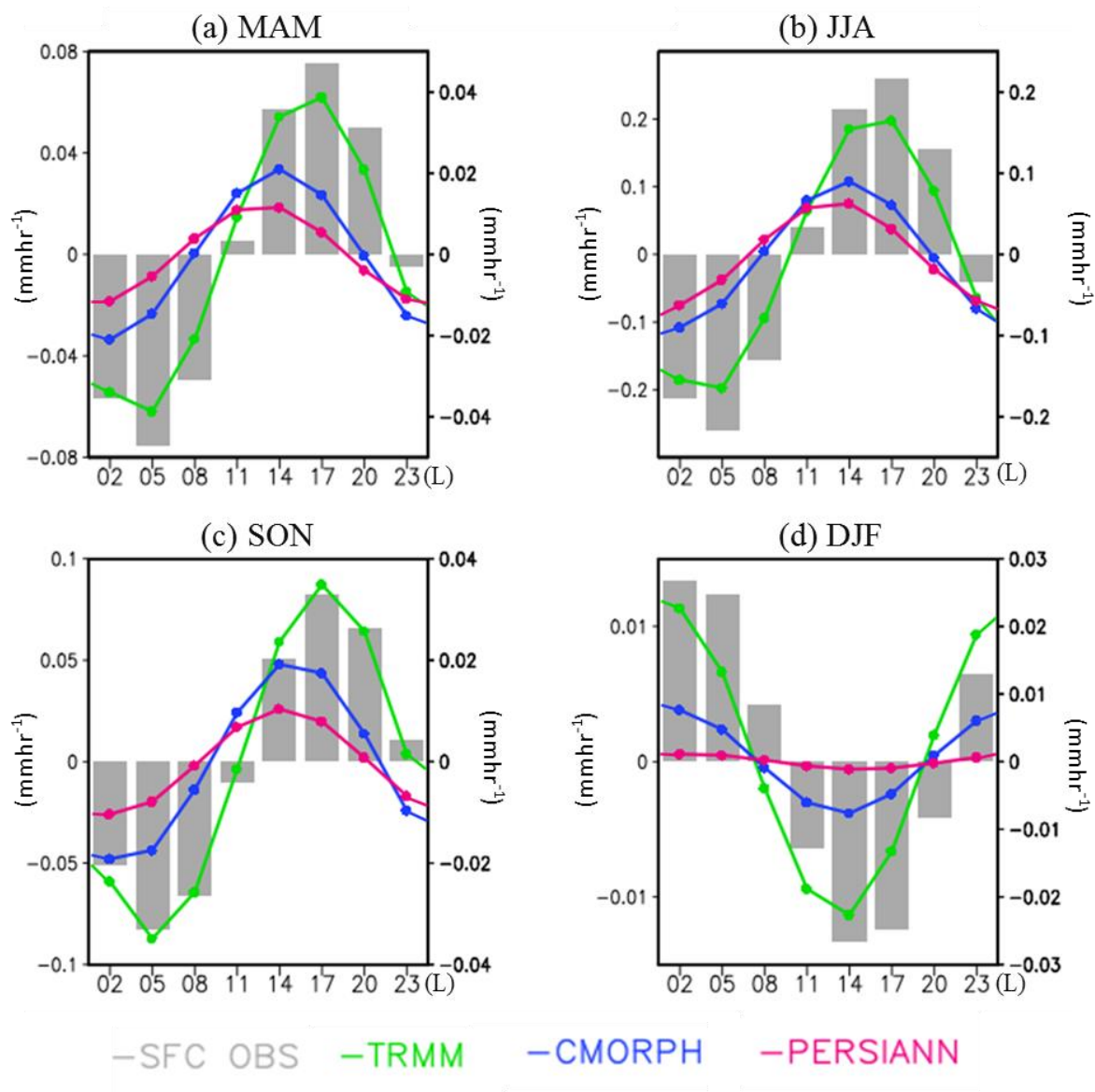
圖 8 類似圖 6，但為日周期變化分量之比較。單位為 \text{mm hr}^{-1} 。
