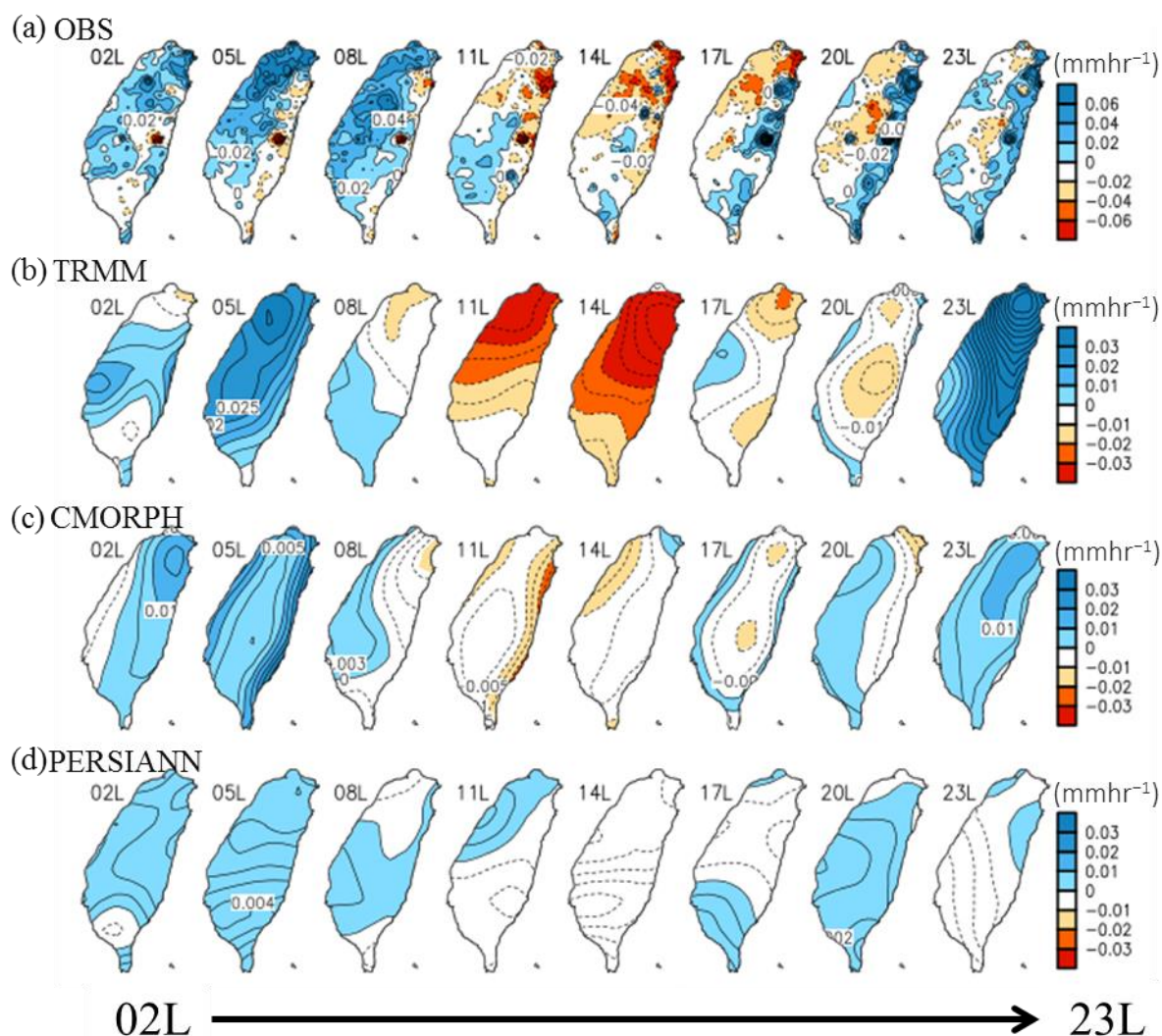
圖 5 類似圖 2，但為冬季降雨日變化量之時間、空間變化。單位為 \text{mm hr}^{-1} 。
