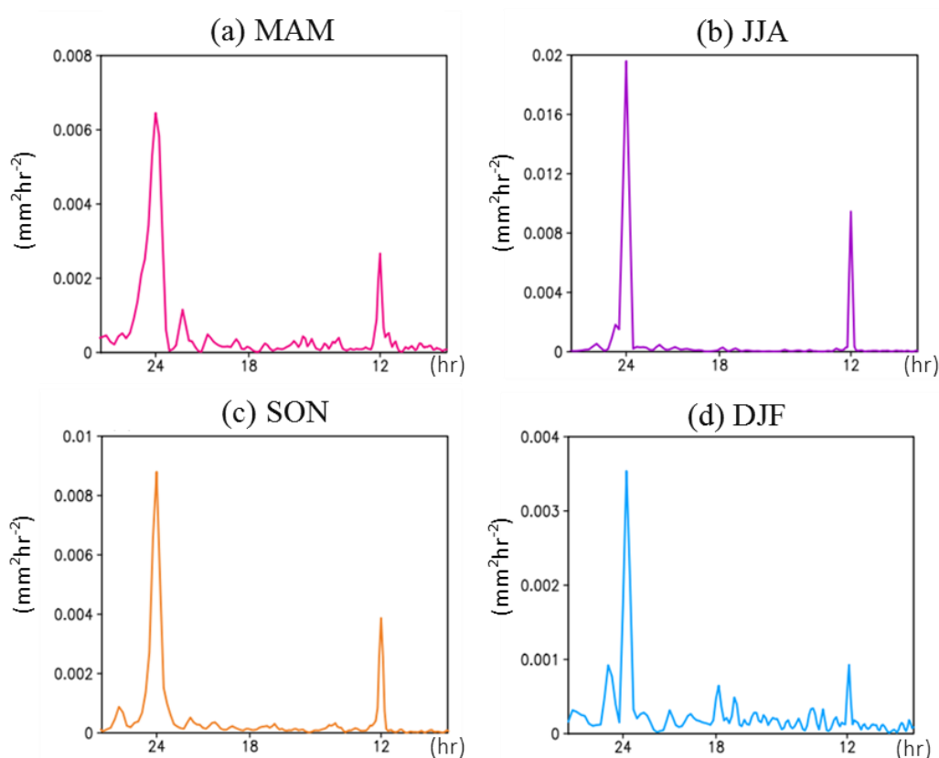
圖 7 針對圖 6 中，地面觀測區域平均後之臺灣降雨每 3 小時變化，所做的波譜分析。(a)春季(b)夏季(c)秋季(d)冬季。橫軸代表振盪周期，縱軸為降雨的振幅平方，單位為 \text{mm}^2 \text{hr}^{-2} 。
