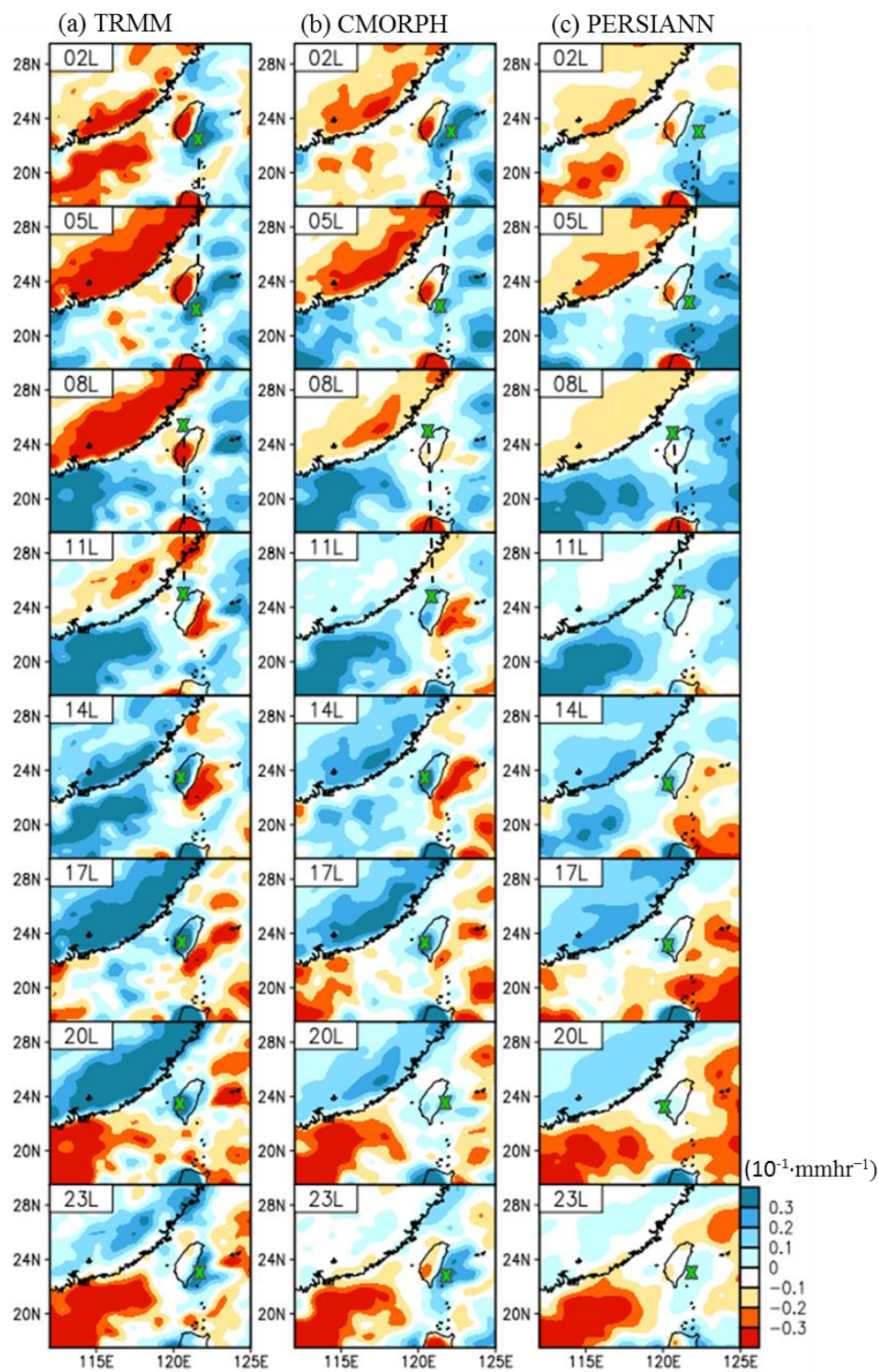
圖 12 類似圖 10，但為秋季降雨日周期水平空間分布。單位為 10^{-1} \text{ mm hr}^{-1} 。
