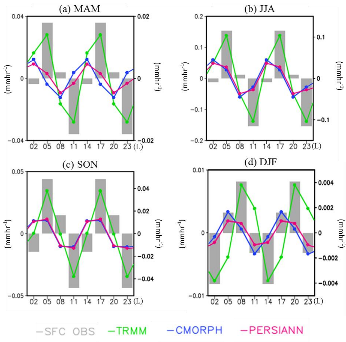
圖 9 類似圖 6，但為半日周期變化分量之比較。單位為 \text{mm hr}^{-1} 。
