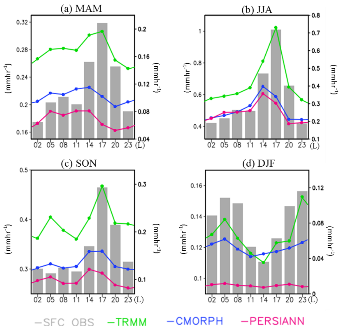
圖 6 區域平均後之臺灣降雨每 3 小時變化。(a)春季(b)夏季(c)秋季(d)冬季。左縱軸表示地面觀測資料(灰柱)雨量值，右縱軸表示衛星資料雨量值(綠線為 TRMM，藍線為 CMORPH，紅線為 PERSIANN)，單位為 \text{mm hr}^{-1} 。
