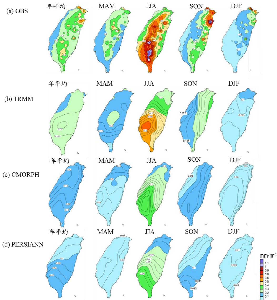
圖 1 臺灣年平均及四季氣候平均場降雨水平空間分布。(a)為地面觀測資料，(b)-(d)為三組衛星觀測資料：(b) TRMM (c) CMORPH 及(d) PERSIANN。色標如圖所示，單位為 \text{mm} \cdot \text{hr}^{-1} 。
