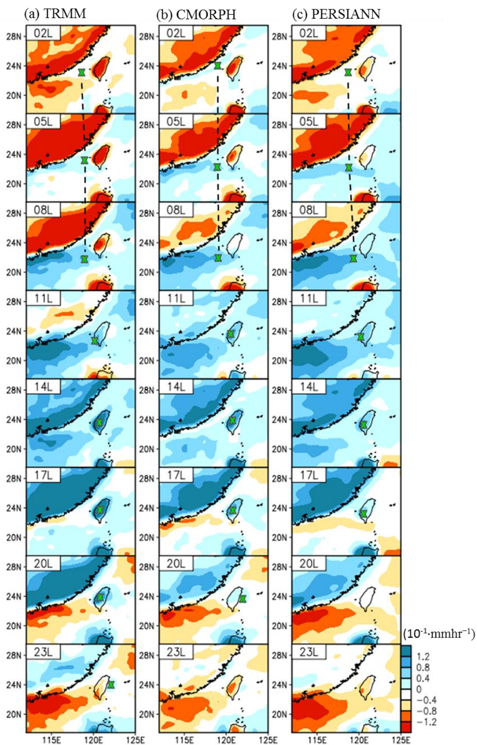
圖 11 類似圖 10，但為夏季降雨日周期水平空間分布。單位為 10^{-1} \text{ mm hr}^{-1} 。
