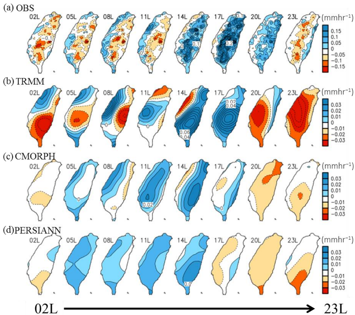
圖2 春季降雨日變化量之時間、空間變化。(a)為地面觀測資料，(b)-(d)為三組衛星觀測資料：(b) TRMM (c) CMORPH 及(d) PERSIANN。色標如圖所示，時間為當地時間 L，單位為 \text{mm hr}^{-1} 。
