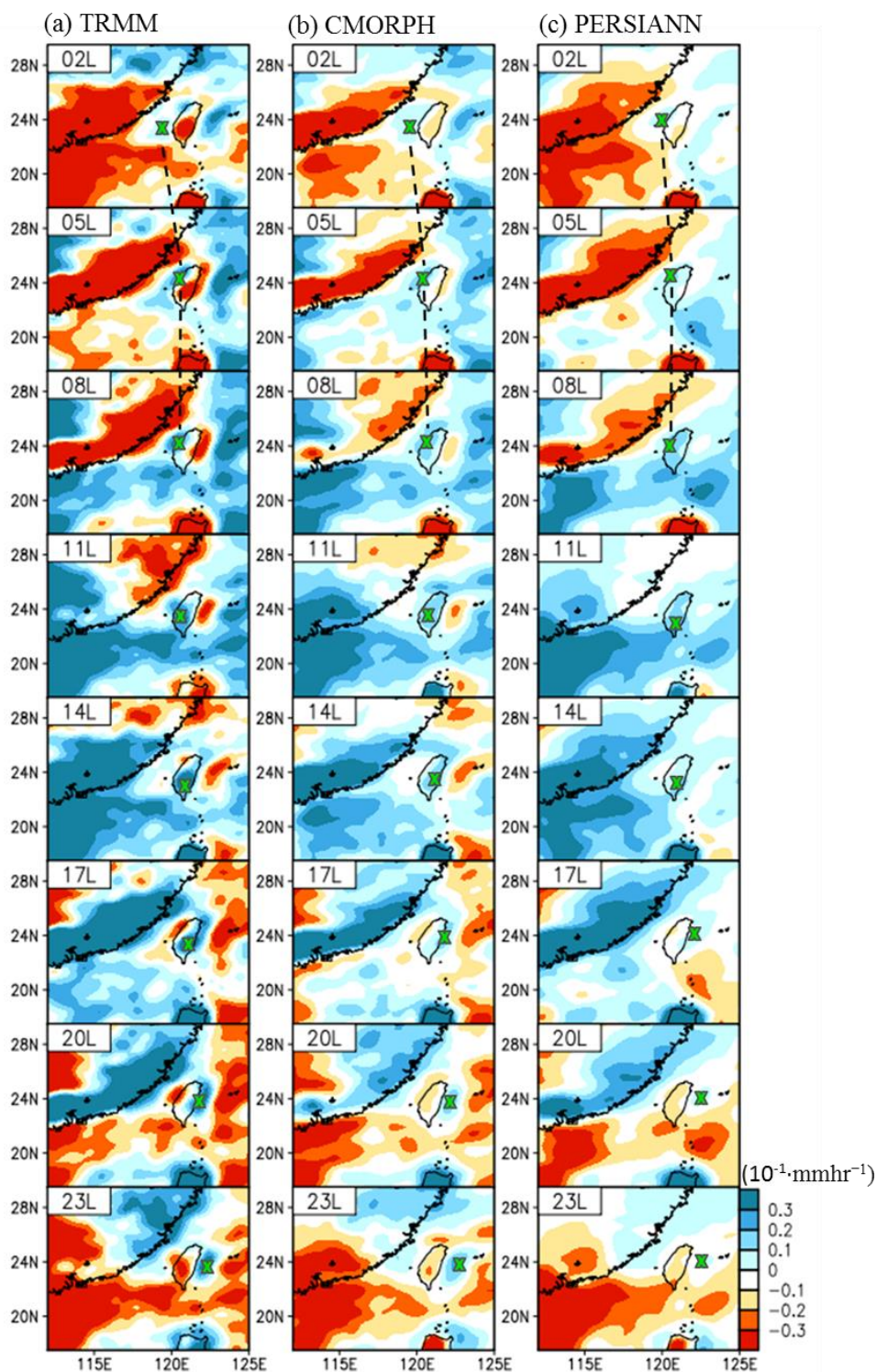
圖 10 春季降雨日周期水平空間分布。(a) TRMM (b) CMORPH 及 (c) PERSIANN。色標如圖所示。綠色 x 之標示，代表影響臺灣降雨之主要雨帶位置，黑色虛線代表文中所提之清晨雨帶移動之連線，單位為 10^{-1} \text{ mm hr}^{-1} 。
