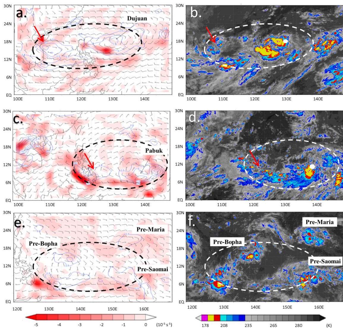
圖2 (a與b) 2009年9月2日1800UTC之(a)NCEP-FNL 850hPa風場(m/s, 風標)、輻散場( 10^{-5}\text{s}^{-1} , 如左下色階)、及渦度場(等值線, 10^{-5}\text{s}^{-1} )與(b)紅外線衛星雲圖(K, 如右下色階)。圖中粗虛線約略標示季風環流圈之位置；圖(a)中黑色標籤(紅色箭頭)指出形成於季風環流圈中颱風(未發展之熱帶擾動)，圖(b)白點為根據圖(a)所標記之系統環流中心。(c與d)同(a與b)但為2001年8月11日0600UTC, Pabuk颱風所形成於之季風環流圈。(e與f)同(a與b)但為2006年8月2日0600UTC, Bopha颱風及 Saomai颱風所形成於之季風環流圈。
