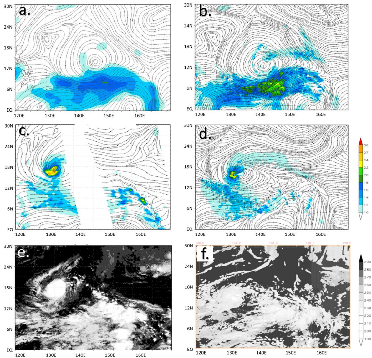
圖 4 WRF 模式模擬結果之校驗。(a、c、及 e) 為重分析與觀測資料，(b、d、及 f) 為 WRF 模式模擬結果。(a) 2004 年 6 月 22 日 0000UTC 之 NCEP-FNL 850 hPa 風場 (m/s，右側色階) 及流線場。(c) 2004 年 6 月 23 日 1200UTC 之 QuikSCAT 海平面風場 (m/s，右側色階) 與流線場。(e) 2004 年 6 月 23 日 1200UTC 之 IR1 雲頂溫度 (K，右下色階)。(b、d、及 f) 如 (a、c、及 e) 但為對應時間 (模式模擬 24 小時與 60 小時) 之 WRF 模擬結果。
