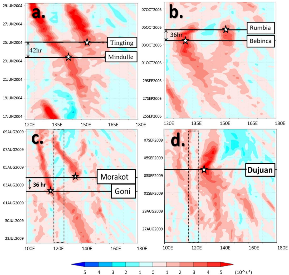
圖 3 (a) 2004 年 Mindulle 颱風及 Tingting 颱風形成期間之 850hPa 緯向平均 ( 5^{\circ}\text{N} \sim 20^{\circ}\text{N} ) 渦度場 ( 10^{-5}\text{s}^{-1} ，如左下色階) 之哈默圖，X 軸為經度、Y 軸為時間。(b) 同(a)，但為 2006 年 Bebinca 颱風及 Rumbia 颱風形成期間。(c) 同(a)，但為 2009 年 Goni 颱風及 Morakot 颱風形成期間。(d) 同(a)，但為 2009 年 Dujuan 颱風形成期間。圖中之星號與黑線標記颱風形成之時間與經度，雙箭頭標記兩颱風形成時間之差異，虛線方框為台灣與菲律賓地形所在之範圍。
