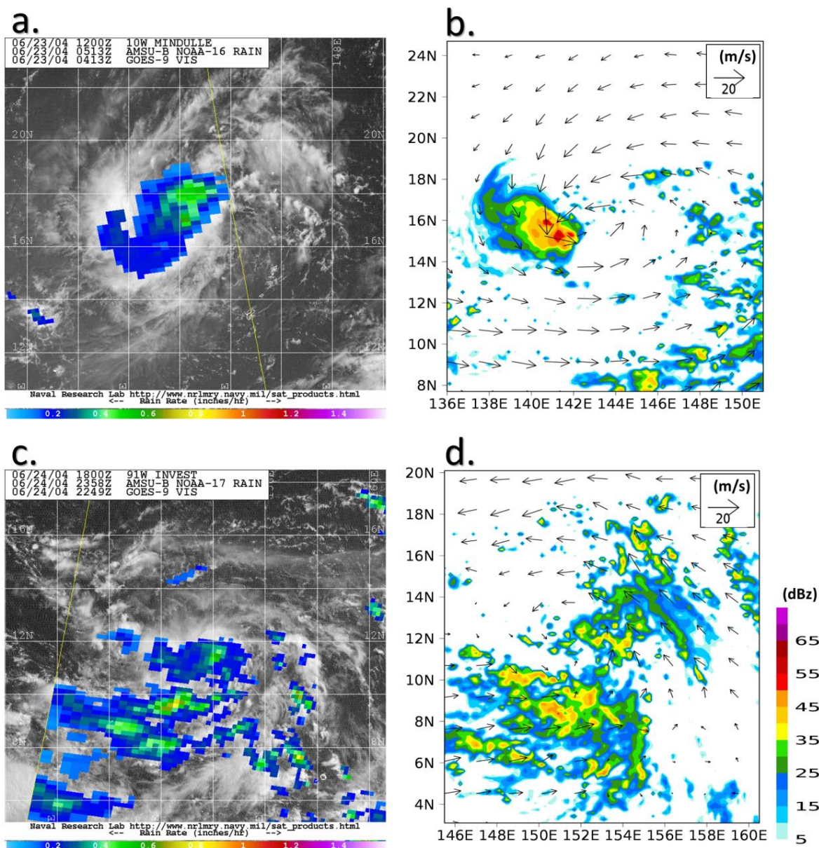
圖 7 (a) 2004 年 6 月 23 日 0513UTC (Mindulle 颱風形成參考點) 之 AMSU 微波頻道衛星觀測之降雨率與紅外線衛星雲圖 (取自美國海軍實驗室颱風網頁: http://www.nrlmry.navy.mil/TC.html )。(b) 對應時間之 WRF 模式模擬雷達迴波 (dBZ, 如右下色階) 與地面風場 (如圖右上風標)。(c 與 d) 同 (a 與 b), 但時間為 2004 年 6 月 24 日 2358UTC (Tingting 颱風形成參考點), 另須注意 (d) 圖為較 (c) 圖晚 3 小時之模擬結果。
