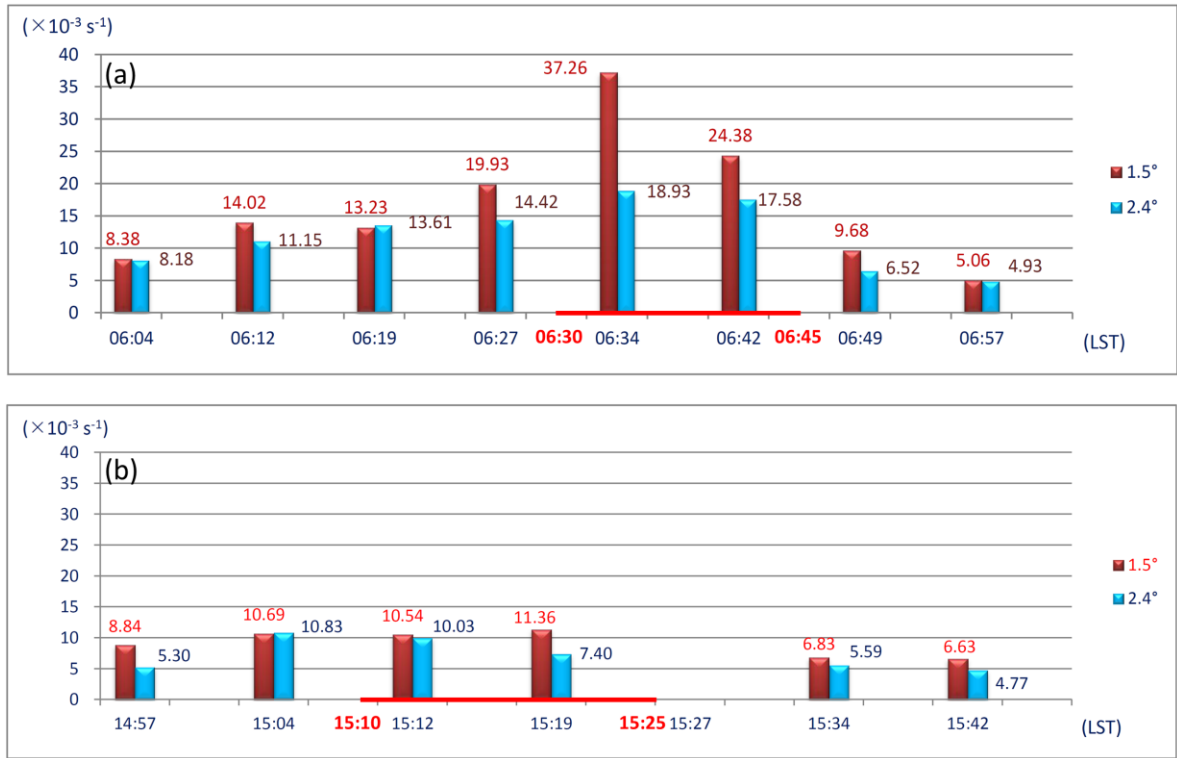
圖 18 風切渦度隨時間變化之分布圖(a) 2015 年 7 月 20 日臺南新化迷你超胞龍捲風事件（紅色粗線代表發生時間 0630~0645 LST）、(b) 2015 年 5 月 24 日臺南下營龍捲風事件（發生時間約為 1510~1525 LST）。其中，紅色直條圖代表仰角 1.5°、藍色直條圖代表仰角 2.4°之風切渦度值 (\times 10^{-3} \text{ s}^{-1}) 。
