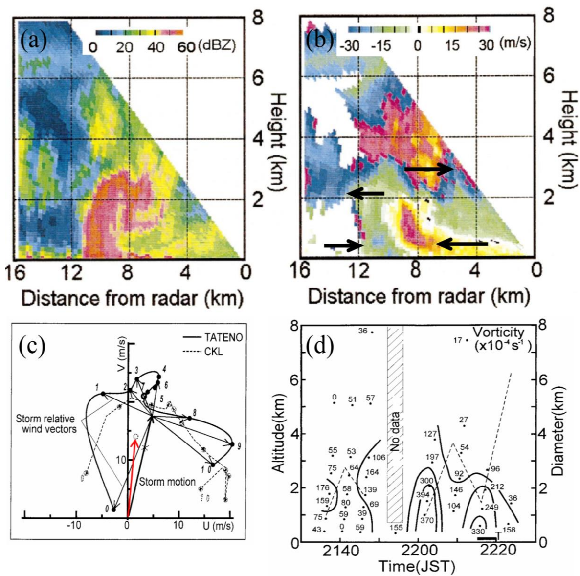
圖 4 激發龍捲風之迷你超大胞的(a) RHI 回波(dBZ), (b) RHI 徑向速度 ( \text{m/s} ), 黑色箭頭 (修改原文箭號大小及粗細) 為相對於雷達之風向。(c)風徑圖, 紅色粗箭頭 (依原圖加繪) 為環境場之平均風向量、黑色粗箭頭為迷你超大胞移動向量、黑色細箭頭為迷你超大胞相對風向量。(d)迷你超大胞垂直渦度隨時間與高度之變化圖。(取自 Suzuki et al., 2000, Fig.6, Fig.12, Fig.13c, and Fig.13d)
