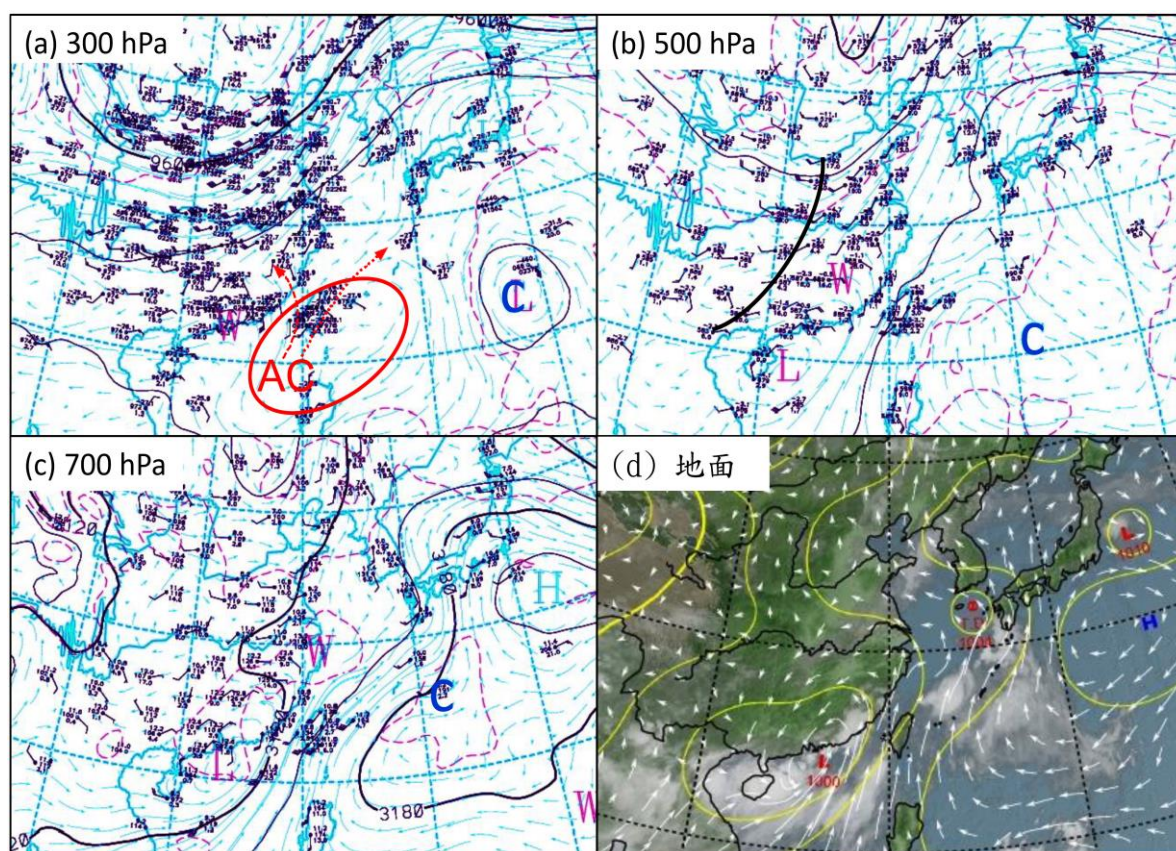
圖 5 2015 年 7 月 20 日 0800LST (a) 300 hPa、(b) 500 hPa、(c) 700 hPa 中央氣象局天氣分析圖，分別疊加 300 hPa、500hPa、700hPa NAVGEM 分析風場，其中，黑色實線為等高線（間距為 30 gpm），紫紅色虛線為等溫線（間距為 3°C），藍色箭頭代表風向及風速，L 為低壓、H 為高壓、C 為冷心、W 為暖心，紅色空心圓為反氣旋式環流(AC)位置，紅色虛線箭頭代表該區風向；(d)中央氣象局地面天氣圖疊加紅外線雲圖及 925 hPa NAVGEM 分析風場，白色箭頭代表風向及風速。
