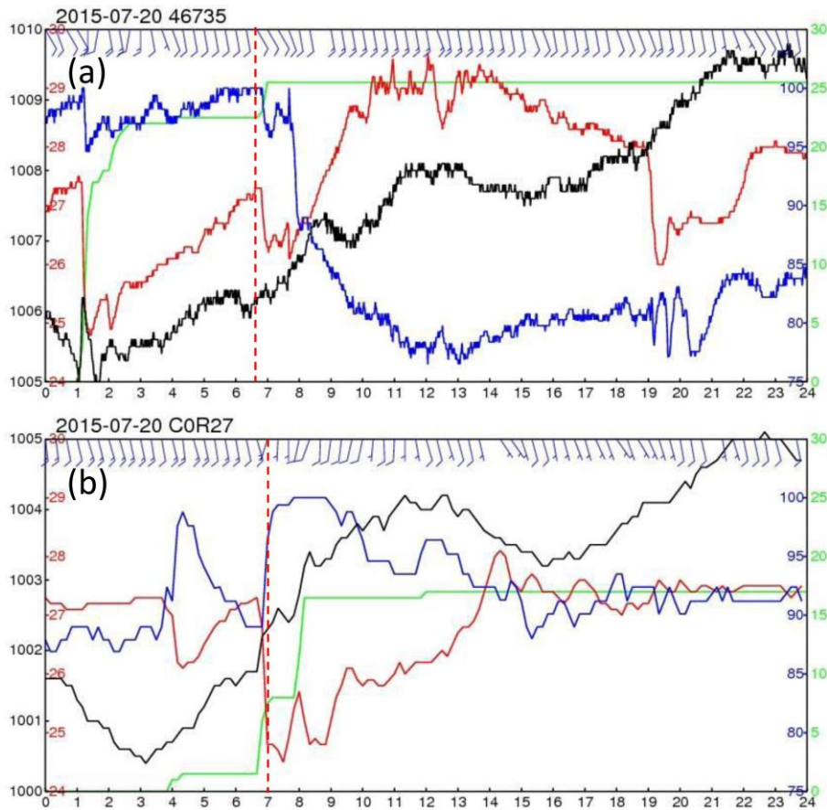
圖 11 2015 年 7 月 20 日(a)澎湖站(46735)、(b)琉球嶼站(C0R27)觀測資料，黑色線代表氣壓(hPa)、紅色線代表氣溫( ^{\circ}\text{C} )、藍色線代表相對濕度(%)、綠色實線代表累積雨量(mm)，以及風標長桿與短桿分別代表風速 5 \text{ m s}^{-1} 與 2.5 \text{ m s}^{-1} 。紅色虛線為陣風鋒面通過時產生之風向轉變。
