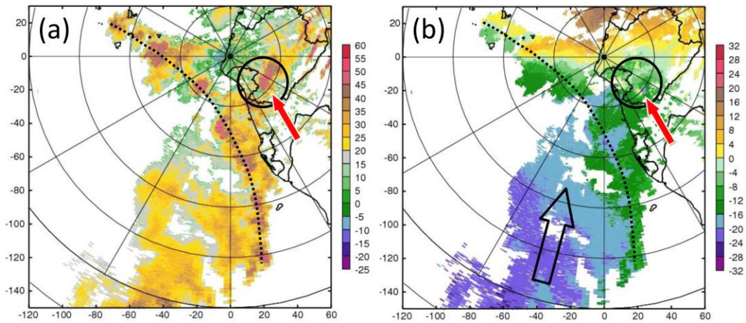
圖 10 2015 年 7 月 20 日 0627 LST 七股雷達於 1.5°仰角 PPI 之(a)回波(dBZ)、(b)徑向速度( \text{m s}^{-1} )。座標軸單位為公里，原點位置為七股雷達站，黑色實線弧線距離為 30 km，黑色虛線為弧形對流雲系所在位置，黑色空心圓為中尺度氣旋所在位置，紅色箭頭各標示鉤狀回波與正負徑向速度區，黑色空心箭頭代表較強入流區。
