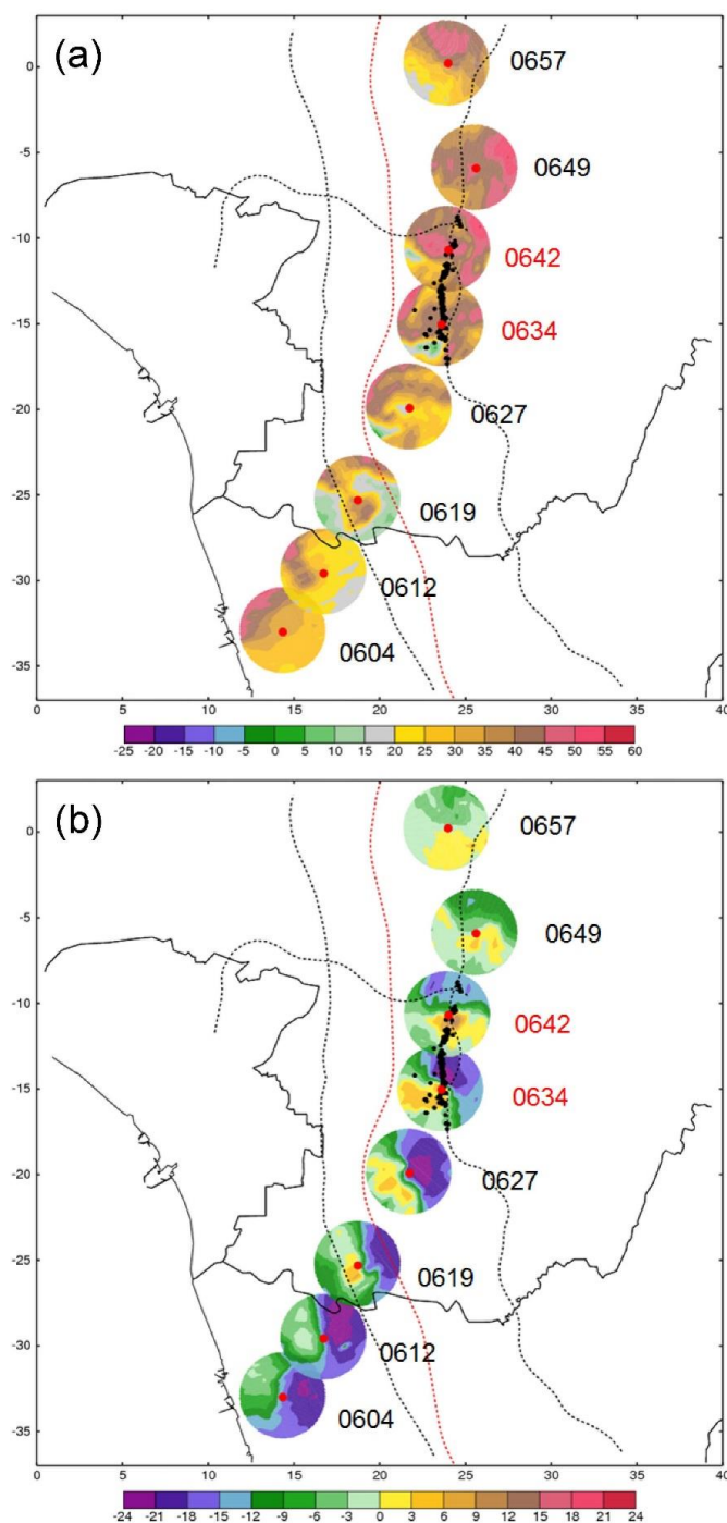
圖 14 2015 年 7 月 20 日 0604 至 0657 LST (每 7.5 分鐘) 七股雷達於 1.5^\circ 仰角 PPI 觀測到中尺度氣旋伴隨龍捲風發生前、發生時及發生後之(a)回波(單位: dBZ)、(b)徑向速度(單位: \text{ms}^{-1} )變化一覽圖。紅點為中尺度氣旋中心, 黑色點位為龍捲風災損軌跡, 黑色點線為國道 1 (左) 與國道 3 (右), 紅色點線為高鐵, 黑色實線為縣市邊界; 0630~0645 LST 為龍捲風大約生成維持時間, 故 0634 與 0642 LST 以紅字標示, 其餘以黑字標示。
