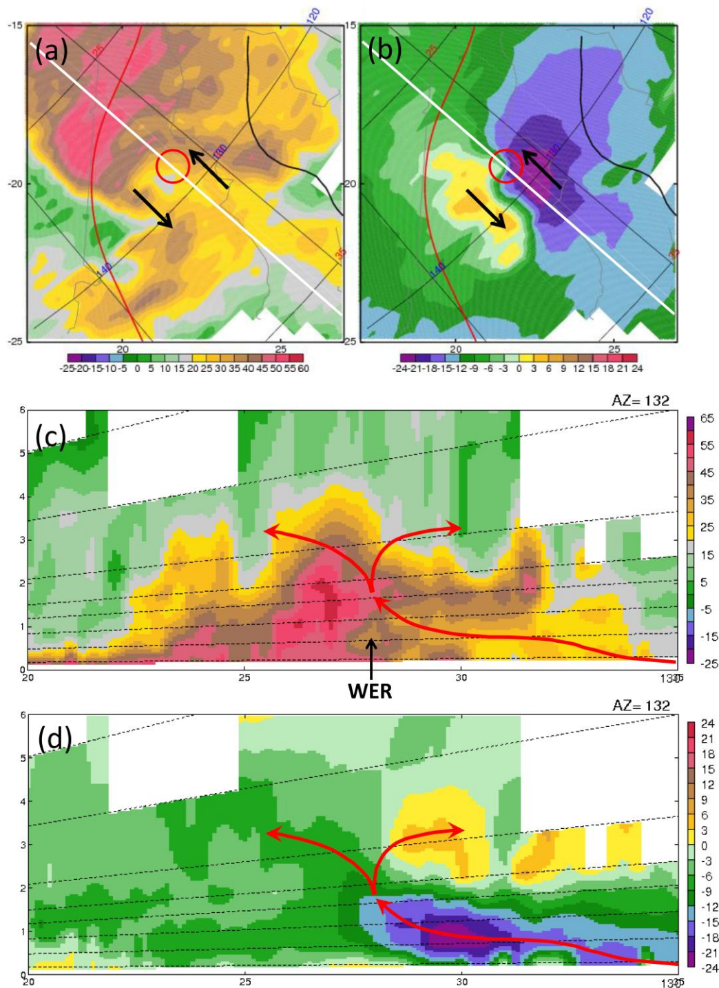
圖 15 2015 年 7 月 20 日 0627 LST 七股雷達站於 1.5° 仰角之 (a) PPI 回波 (單位: dBZ)、(b) PPI 徑向速度 (單位: \text{m s}^{-1} )，黑色箭頭為徑向速度場定出之風向及紅色空心圓為中尺度氣旋所在位置，白色實線為選定之 132° 方位角。於 132° 方位角之 (c) RHI 回波 (單位: dBZ)、(d) RHI 徑向速度 (單位: \text{m s}^{-1} )，紅色箭頭代表入流及輻散位置，WER 為弱回波區。
