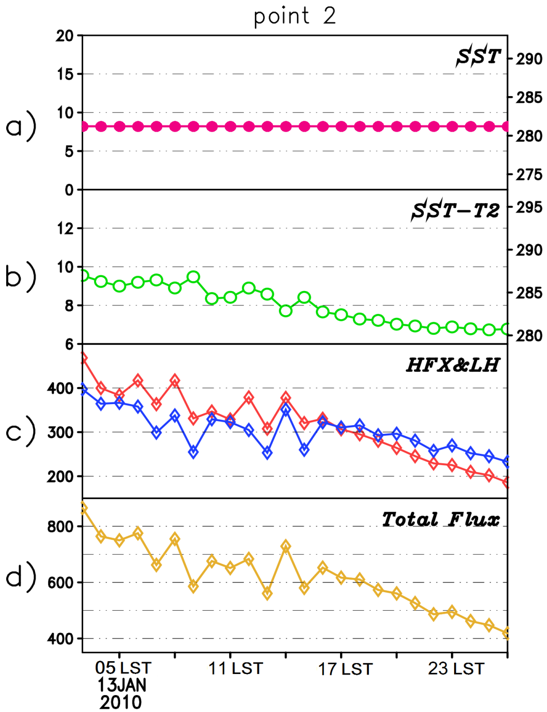
圖 17 同圖 16，但為綠色實心點 2。
