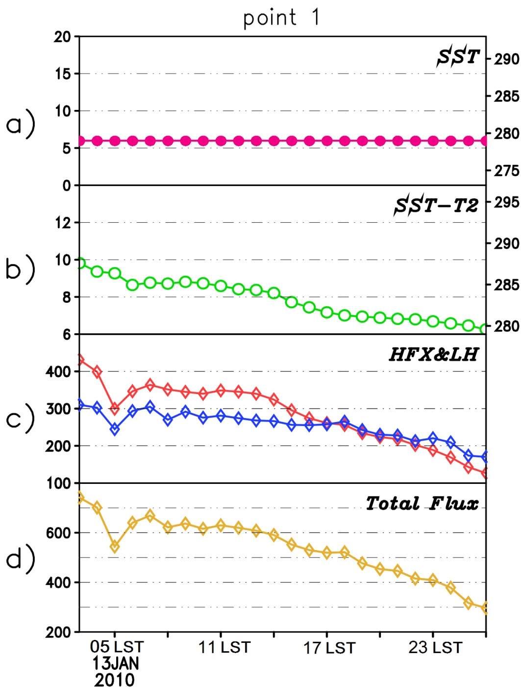
圖 16 圖 10 中綠色實心點 1，2010 年 1 月 13 日 03 LST 至 14 日 02 LST 時間序列圖。(a)海溫、(b)海溫與海面上 2 公尺的氣溫差異、(c)可感熱通量（紅色線）與潛熱通量（藍色線）及(d)總通量（可感熱通量和潛熱通量的總和）。
