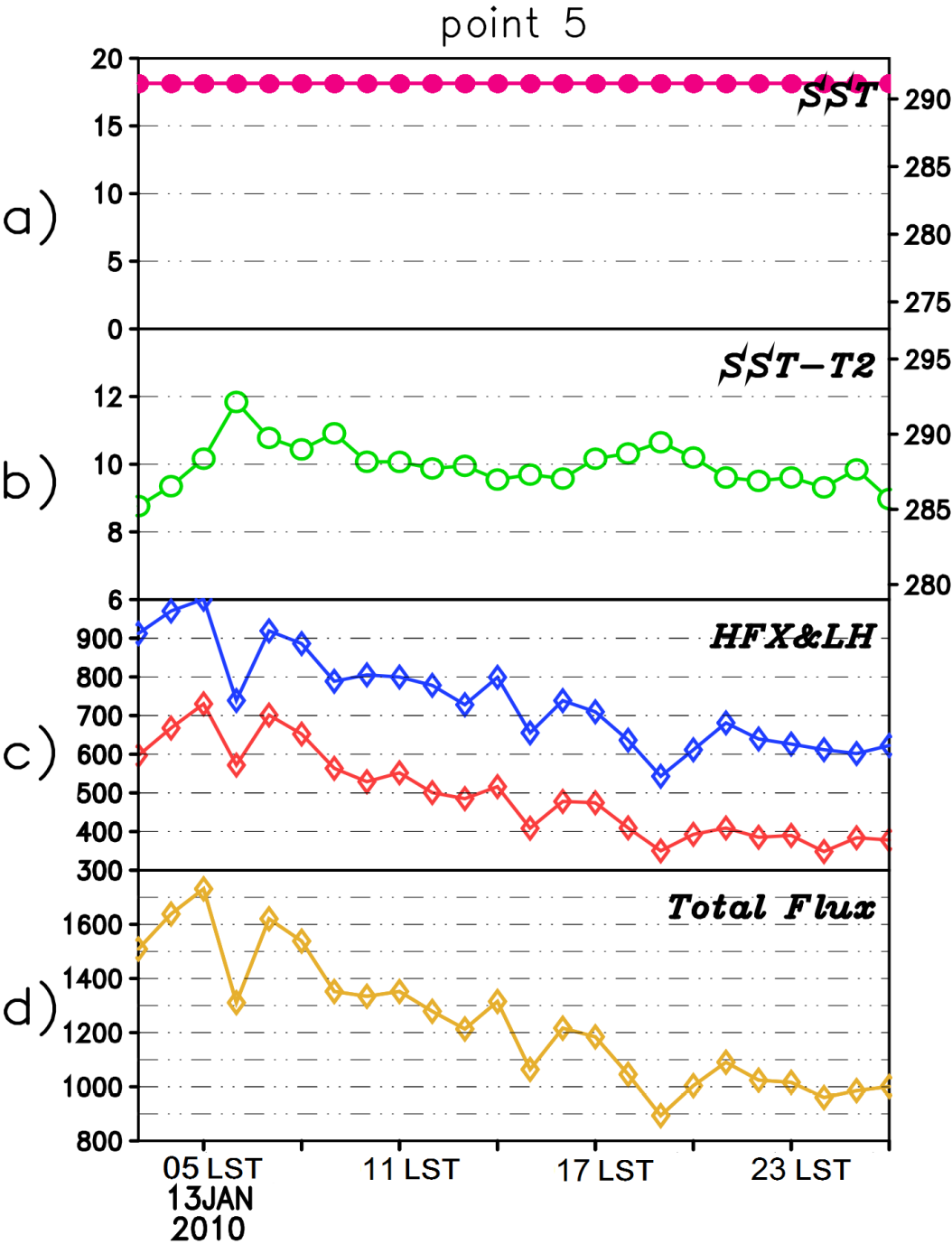
圖 19 同圖 16，但為綠色實心點 5。
