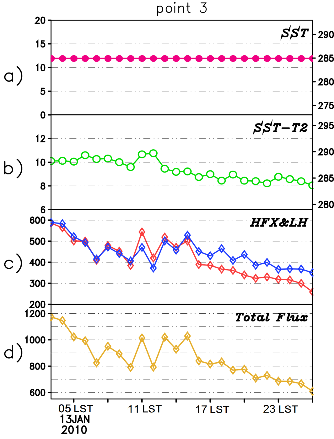
圖 18 同圖 16，但為綠色實心點 3。
