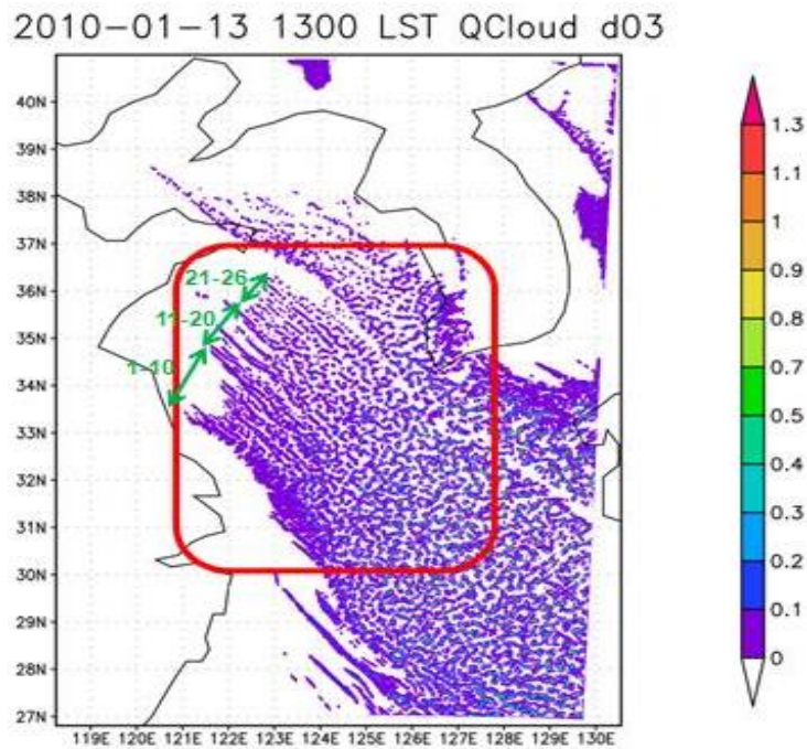
圖 8 模擬時間 2010 年 1 月 13 日 1300 LST，1000 hPa 至 700 hPa 液態水累積圖（顏色對應右方色階，單位為 \text{kg kg}^{-1} ），圖中紅色方框重點分析區域，數字為雲街數量。
