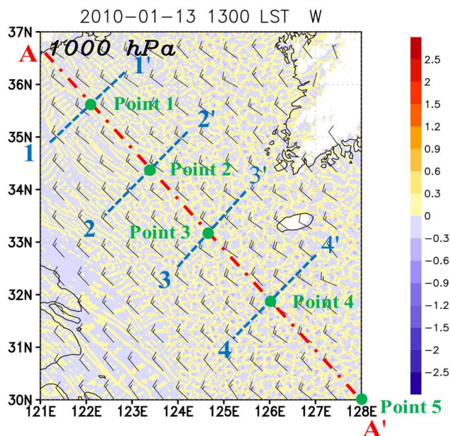
圖 10 同圖 8，但為 1000 hPa 之垂直運動(色階區域，顏色對應右方色階，單位為 \text{m s}^{-1} )、洋面上 1000 hPa 之風標（長、短風標為 10 \text{ m s}^{-1} 、 5 \text{ m s}^{-1} ）與地形（黑色細實線）之合成示意圖。紅色點虛線代表冷空氣上游（A）至下游（A'）的垂直剖面位置，藍色虛線分別代表上游（11'）、中游（22'）、下游（33'及 44'）的垂直剖面位置，綠色實心點 1 至點 5 為挑選代表上、中、下游及更下游特定之分析位置。
