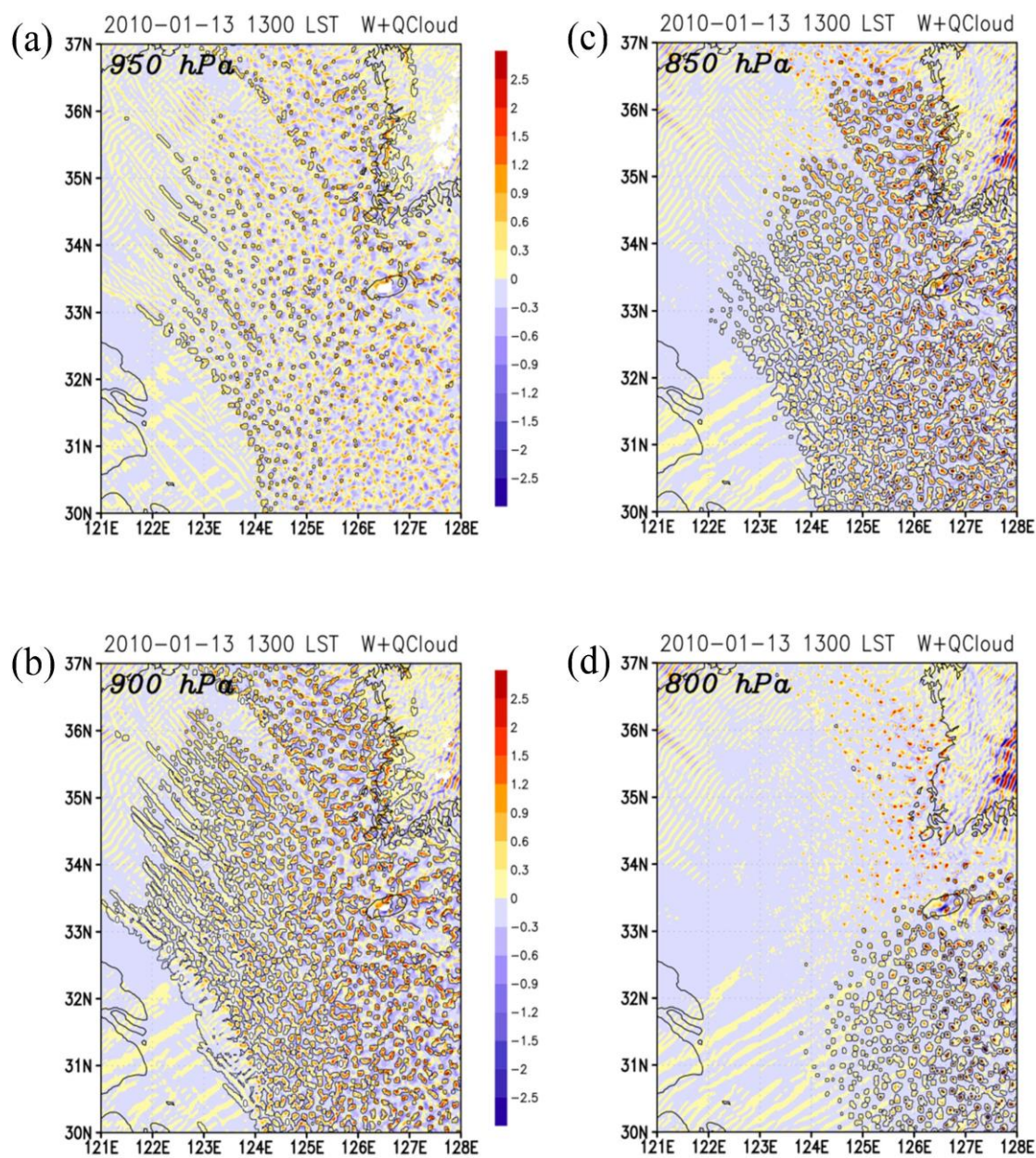
圖 15 1300 LST 垂直運動場（色階， \text{m s}^{-1} ）與液態水（等值線， \text{kg kg}^{-1} ）合成示意圖。(a) 950 hPa、(b) 900 hPa、(c) 850 hPa 及(d) 800 hPa。
