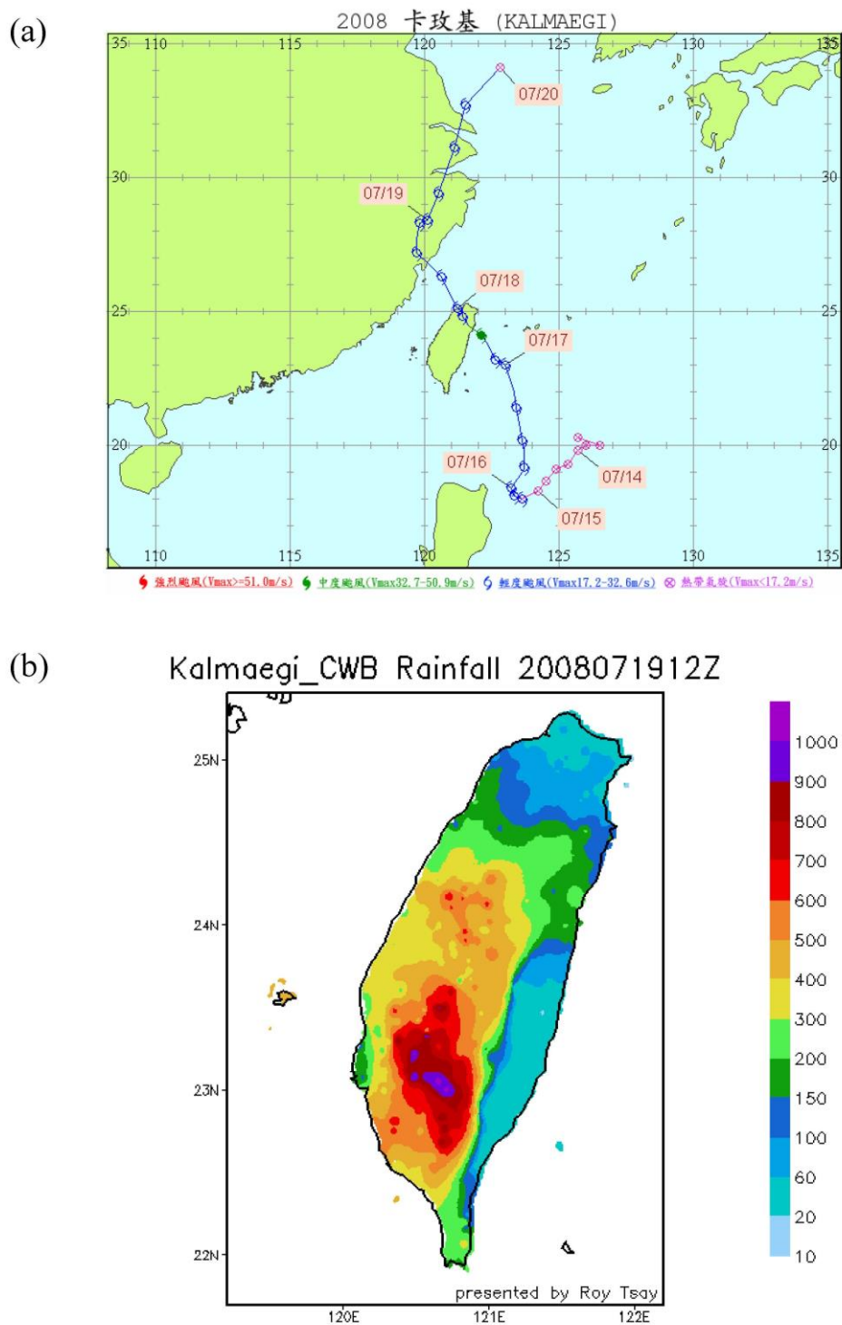
圖 1 (a)卡玫基颱風路徑圖、(b)2008 年 7 月 16 日 0000 UTC 至 19 日 1200 UTC 累積雨量圖 (資料來源：中央氣象局、大氣研究資料庫)。
