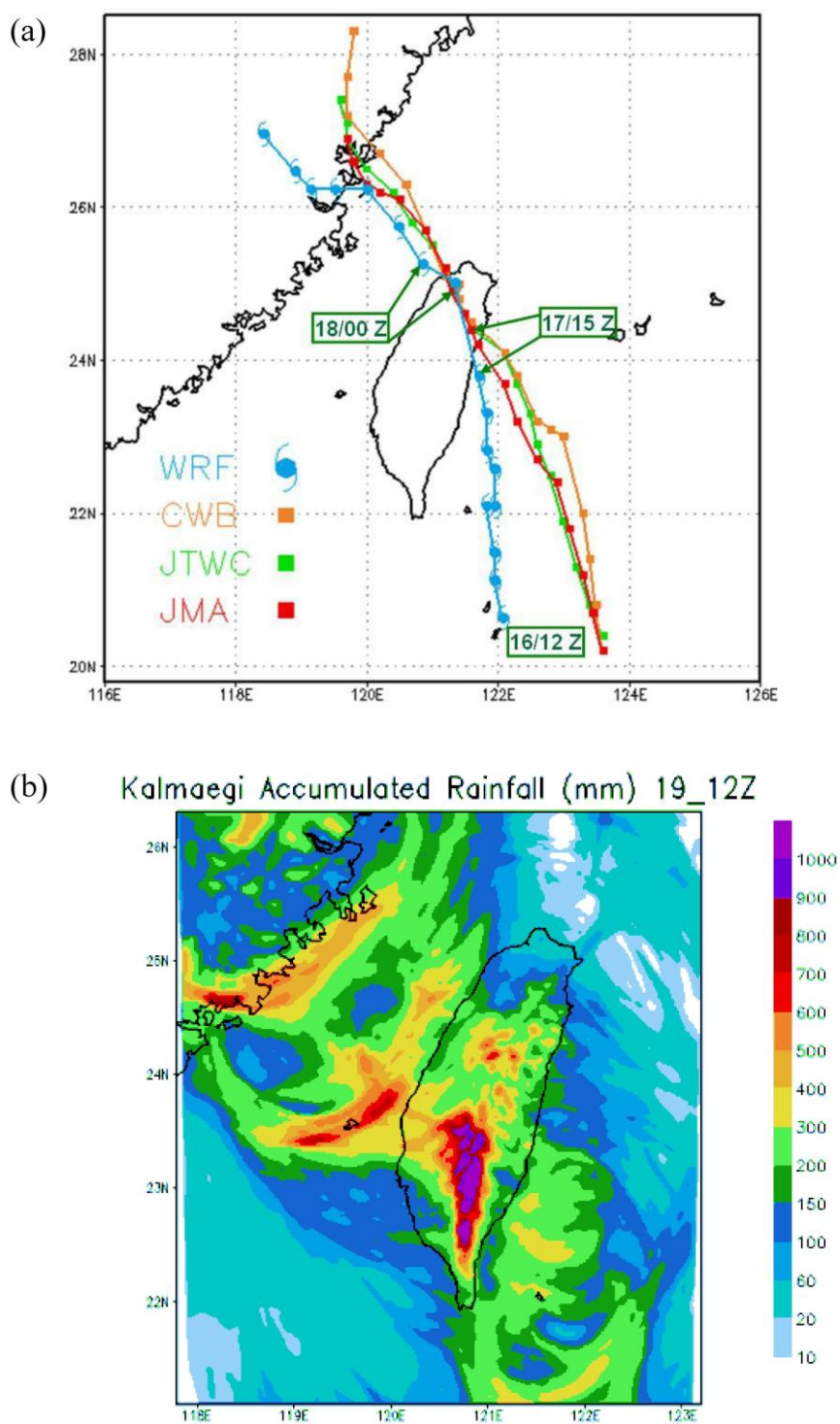
圖 3 (a) 2008 年 7 月 16 日 1200 UTC 至 18 日 1800 UTC 卡玫基颱風路徑圖，間隔為 3 小時，各色圖示分別代表模擬結果(D02)及各作業機構定位路徑、(b) 2008 年 7 月 16 日 0000 UTC 至 19 日 1200 UTC 模擬累積雨量圖(D03)。
