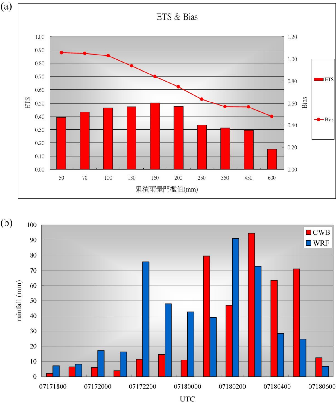
圖 4 (a)模擬降雨(D03)公正預兆得分(直方圖)及偏倚得分(折線圖)、(b)澎湖測站觀測記錄(CWB)與模擬結果(WRF, D03)時雨量直方圖。
