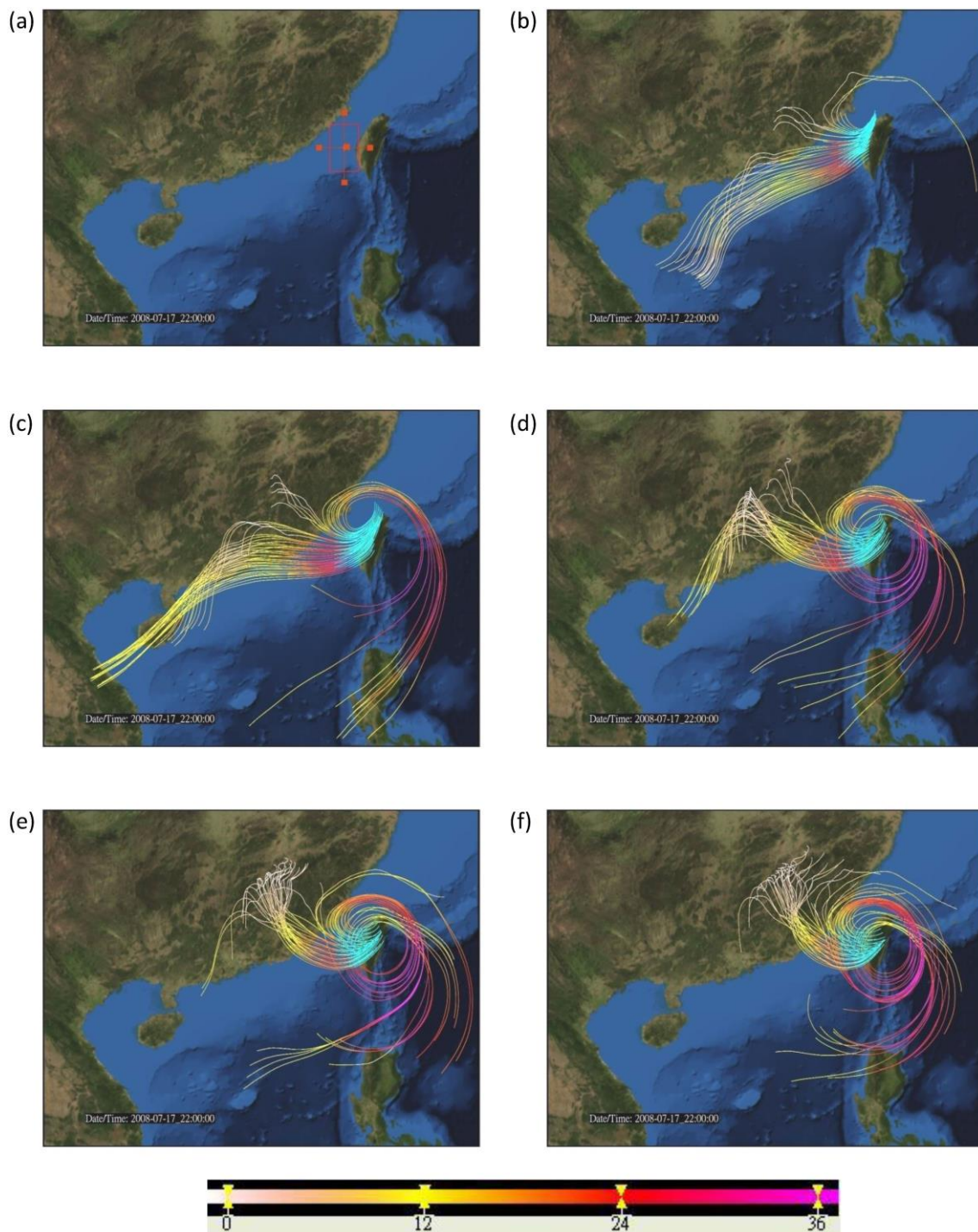
圖 8 (D01)取樣 50 點前、後向積分軌跡疊合圖。積分起始時間為 2008 年 7 月 17 日 2200 UTC，積分間隔為 10 分鐘；淺藍色為前向積分 200 分鐘軌跡線（無風速強度）、其他顏色對應下方風速色階強度（單位為 \text{m s}^{-1} ），為後向積分 2500 分鐘軌跡線。其中(a)表示取樣區域（台灣西側橘色方框），其他各圖取樣高度分別為(b) 469 m、(c) 1523 m、(d) 3016 m、(e) 3982 m、(f) 5035 m。
