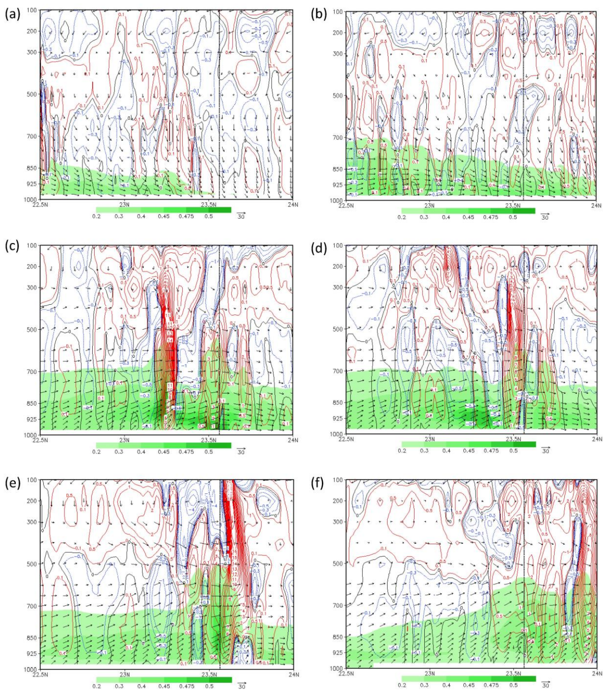
圖 7 (D03) 119.6°E 南北向垂直剖面圖，縱軸為氣壓，單位為 hPa；橫軸為緯度；箭號表水平風，單位為 \text{m s}^{-1} ；等值線表垂直速度，紅色為正值、藍色為負值、黑色為零值線，單位為 \text{m s}^{-1} ；色階表緯向風速與水氣混合比之乘積，單位為 \text{m kg s}^{-1} \text{kg}^{-1} 。時間分別為 2008 年 7 月(a) 17 日 1200 UTC、(b) 17 日 1500 UTC、(c) 17 日 2130 UTC、(d) 17 日 2140 UTC、(e) 17 日 2300 UTC、(f) 18 日 0500 UTC。垂直虛線為澎湖所在緯度(23.6°N)。
