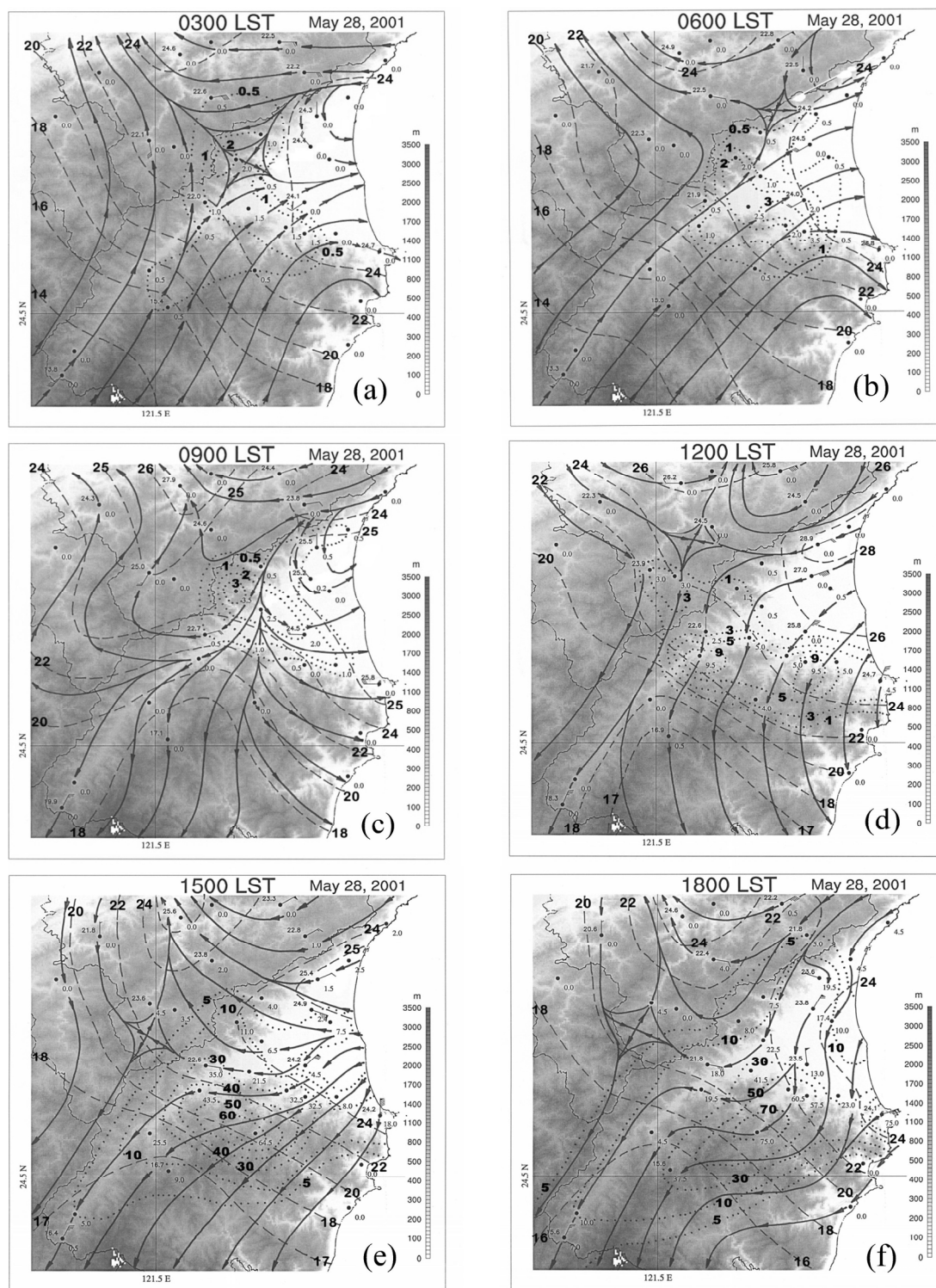
圖8 2001年5月28日(a) 0300、(b) 0600、(c) 0900、(d) 1200、(e) 1500、(f) 1800、(g) 2100及(h) 2400 LST地面中尺度分析。測站左上角為溫度，右下角為3小時降雨量(mm)，風標短桿為 0.25 \text{ ms}^{-1} ，長桿為 0.5 \text{ ms}^{-1} ，三角旗為 2.5 \text{ ms}^{-1} 。虛線為等溫線（以粗體數字表示），點線為等雨量線（以粗體數字表示）。
