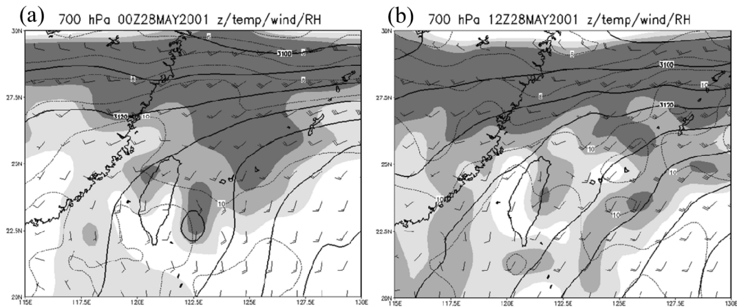
圖4 同圖2,但為700 hPa。
