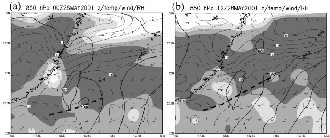
圖3 同圖2,但為850 hPa。
