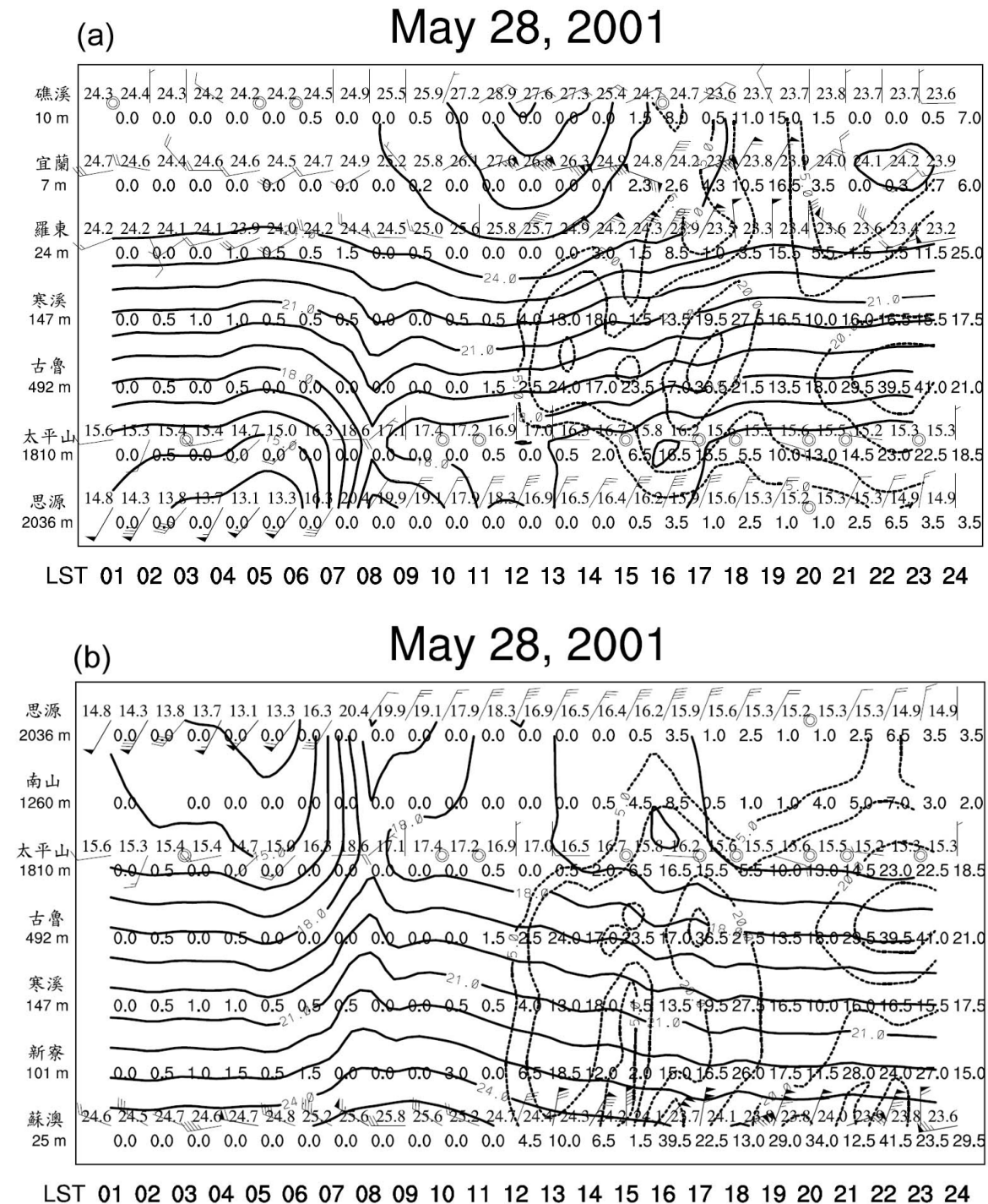
圖9 2001年5月28日0100-2400 LST (a)南北向橫跨主要降雨帶與(b)東西向橫跨主要降雨帶之時空剖面中尺度分析。風標短桿為 0.25 \text{ ms}^{-1} ，長桿為 0.5 \text{ ms}^{-1} ，三角旗為 2.5 \text{ ms}^{-1} 。實線為等溫線（較淡細數字）、點線為等雨量線（較淡細數字）。測站左上方數字為溫度( ^{\circ}\text{C} )，右下方數字為時雨量( \text{mm h}^{-1} )。
