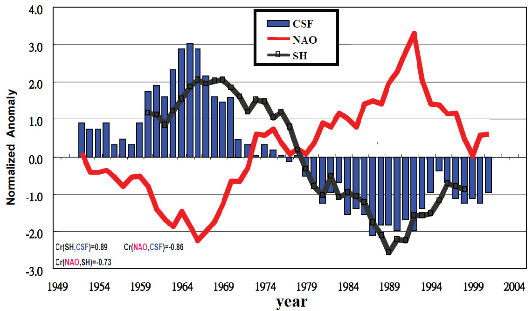
圖 20 臺北寒潮頻率(直方圖)、西伯利亞高壓指標(黑色線)和 NAO(紅色線)之年代際(七年滑動平均)演變。在此，寒潮定義根據中央氣局，每日最低溫小於 10^{\circ}\text{C} 以下稱之；西伯利亞高壓指標為 40^{\circ}\text{N} \sim 60^{\circ}\text{N} ， 80^{\circ}\text{E} \sim 120^{\circ}\text{E} 海平面平均氣壓(Wu and Wang 2002)；NAO 為冬季(DJF)葡萄牙里斯本(Lisbon)與冰島 Stykkisholmur 二測站標準化之地面氣壓的差值。(摘自 Hong et al. 2008)
