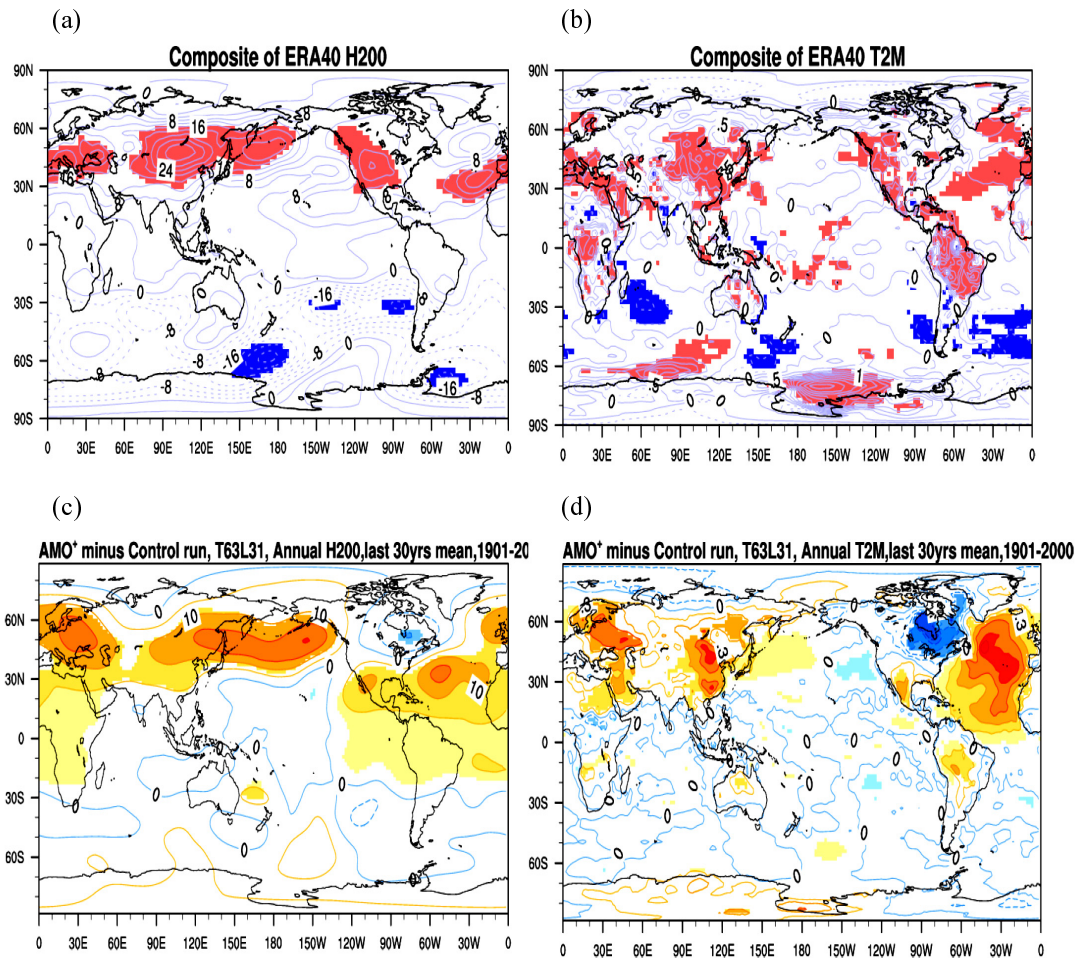
圖5 EAPMO 正相位時的(a) 200hPa 高度與(b) 2m 溫度距平。北大西洋為正海溫距平時，模式模擬的(c) 200hPa 高度與(d) 2m 溫度距平。(摘自 Hsu and Lee 2011)
