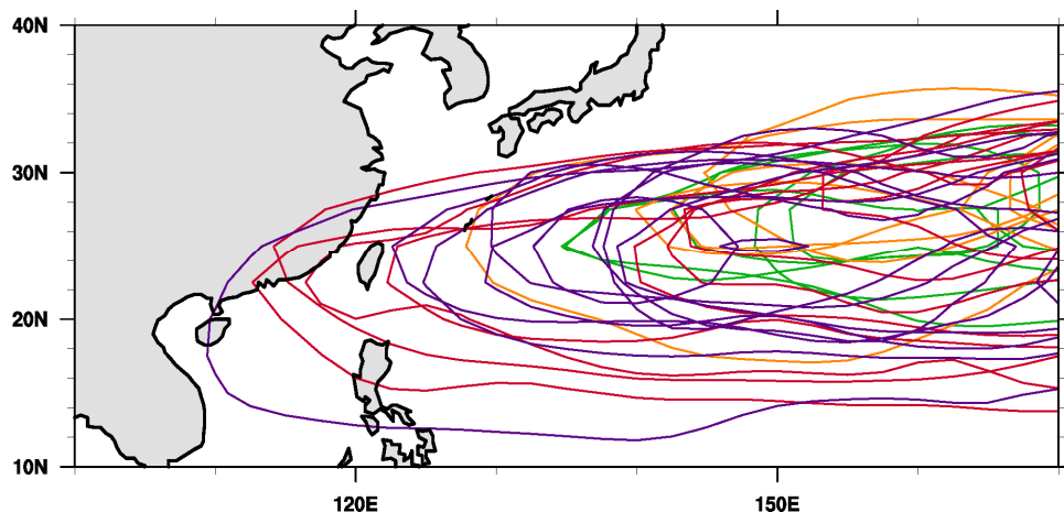
圖 16 1960 年至 1999 年各年夏季平均的 500hPa 高度場 5880m 等值線，綠、橘、紅、紫色分別為 1960 年代、1970 年代、1980 年代、1990 年代。(TCCIP 計畫提供)
