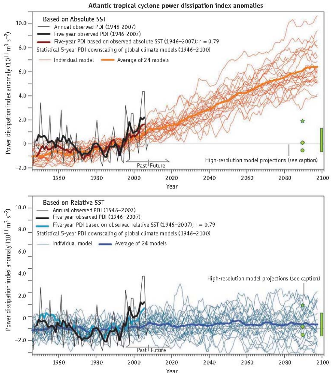
圖 17 大西洋颱風強度(power dissipation index, PDI)在 1946~2007 年期間的變化，包含觀測資料和模式推估； (a)根據海溫的大小 (b)根據海溫的空間分佈（大西洋海溫相對於其他大洋溫度的變化）。 （摘自 Vecchi et al. 2008b）
