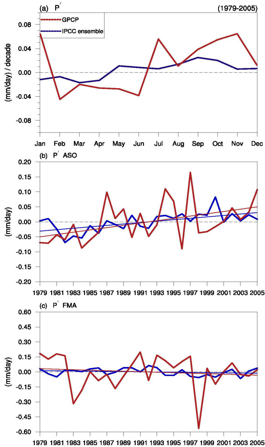
圖 11 北半球熱帶平均降雨在 1979~2005 年期間的季節變化(a)每一個月的變化趨勢，(b)夏季平均的時間序列，(c)冬季平均的時間序列。紅線是衛星觀測資料，藍線是 IPCC 第四次評估報告中的氣候模式平均。 (摘自 Chou et al. 2007, 圖 3)
