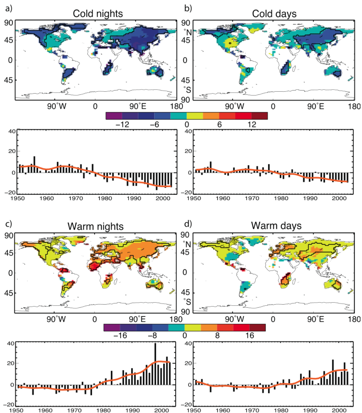
圖 7 極端溫度在 1951~2003 期間各地的變化趨勢和全球時間序列：(a)冷夜 (b)冷晝 (c)暖夜 (d)暖晝。 (摘自 IPCC 第四次評估報告，FAQ3.3 圖 1)
