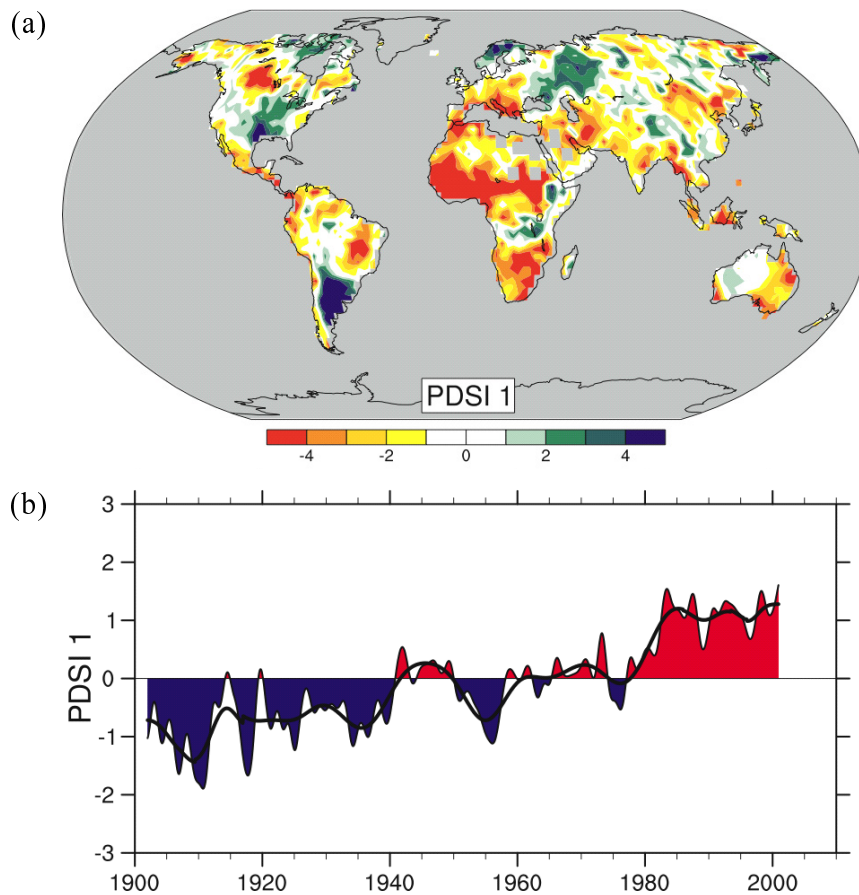
圖6 乾旱指數在1900年~2002年期間的變化趨勢，(a)為空間分佈，(b)為全球平均的時間序列。(摘自 IPCC 第四次評估報告，FAQ3.2，圖1)
