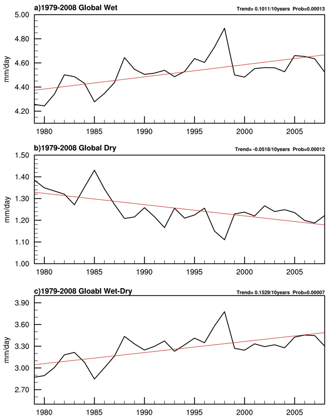
圖 12 全球觀測降雨平均在 1979~2008 年期間的變化：(a)濕季，(b)乾季，(c)濕季減乾季。(Chou and Lan 提供)
