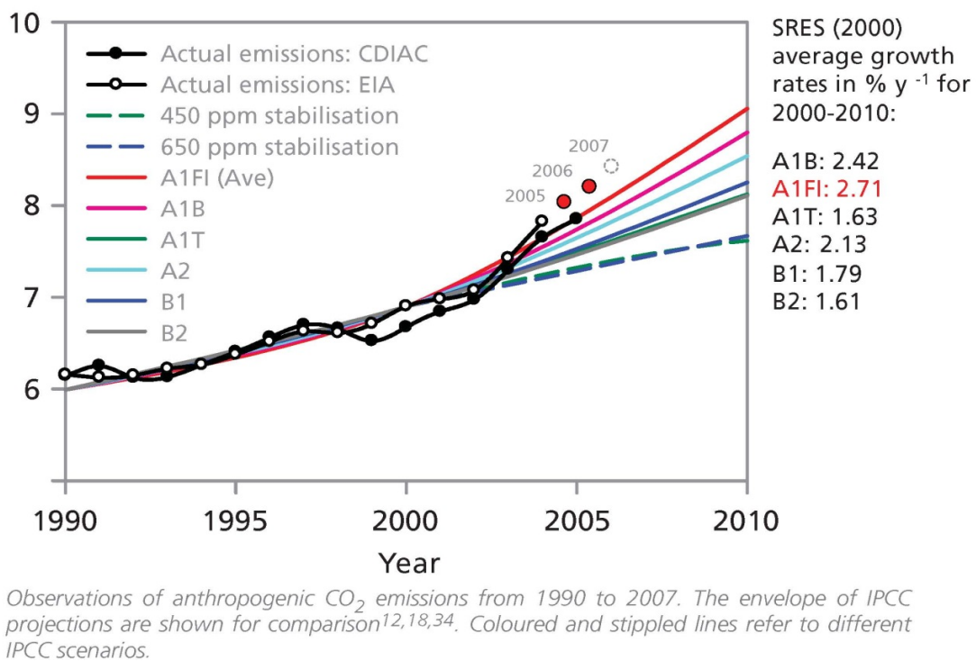
圖 19 二氧化碳在 1990~2007 年期間的排放量。(摘自 Richardson et al. 2009, Box 2)
