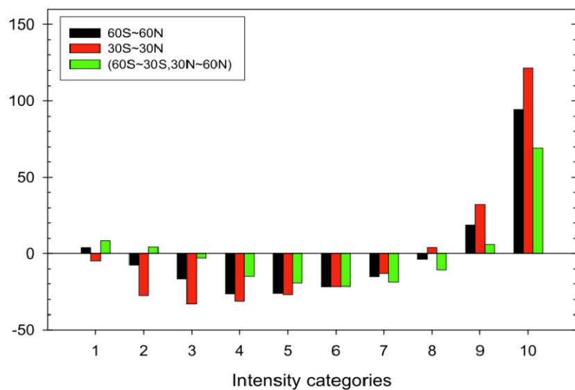
圖 15 降雨強度(ΔP)隨全球溫度(ΔT)之變化圖,紅色為低緯度值(30°S~30°N),綠色為中緯度值(60°S~30°S、30°N~60°N),黑色則為兩者平均值。(Liu et al.提供)
