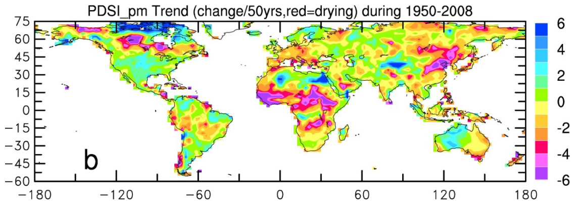
圖 16 全球乾旱指數在 1950~2008 年期間的變化趨勢，紅色區域表示越乾，藍色則是越濕。(摘自 Dai 2010)
