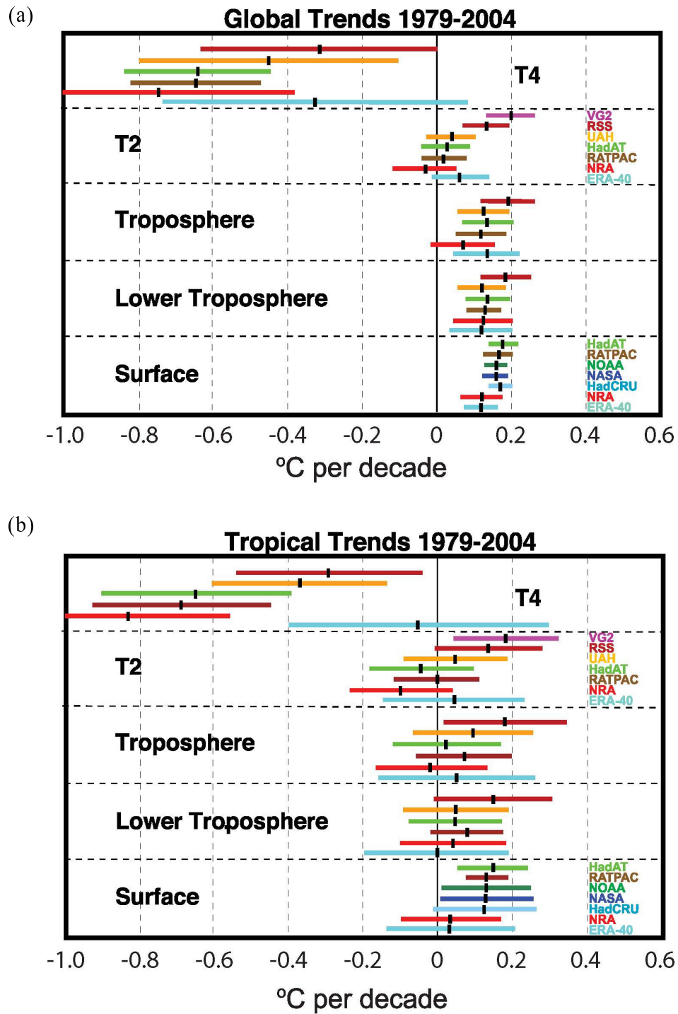
圖2 不同觀測資料中不同高度的溫度在 1979~2004 年期間的線性趨勢。(a)全球平均(b)熱帶平均。圖中 T2 和 T4 分別表示對流層和平流層溫度。(摘自 IPCC 第四次評估報告，圖 3.18)
