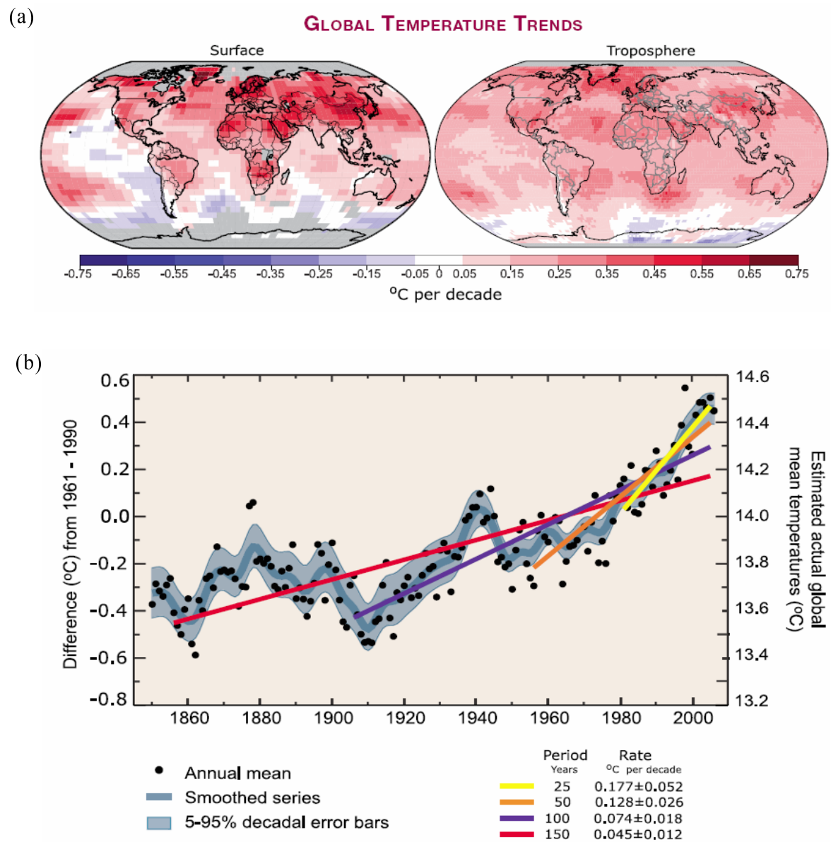
圖 1 全球平均溫度變化與趨勢圖。(a)全球地面（左）和對流層（右）溫度在 1979~2005 年間的變化趨勢。 (b)全球平均地面溫度相較於 1961~1990 年之平均面溫度的變化。 (摘自 IPCC 第四次評估報告，圖 TS.6)
