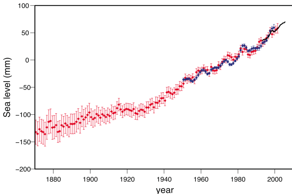
圖 8 全球平均海平面相較於 1961 年至 1990 年之間平均高度的變化。 (IPCC 第四次評估報告，圖 5.13)
