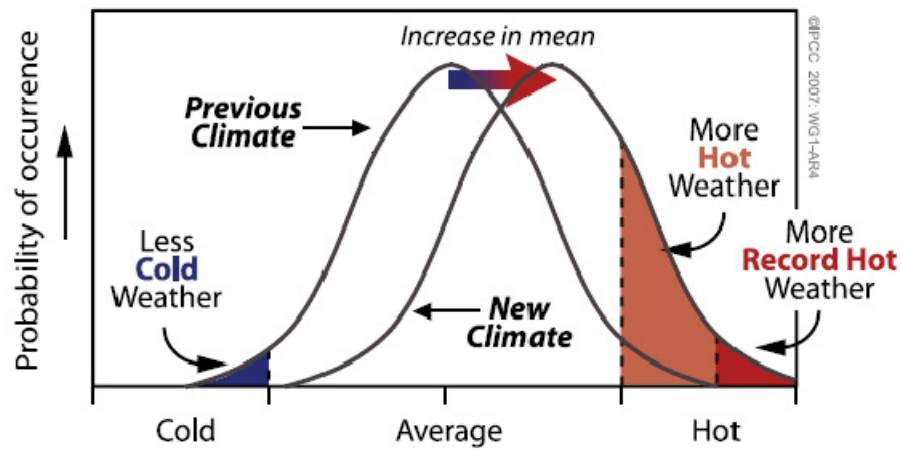
圖5 圖表顯示當溫度分佈為常態分佈時，平均溫度增加對極端氣溫的影響。(摘自 IPCC 第四次評估報告，Box TS.5 圖1)
