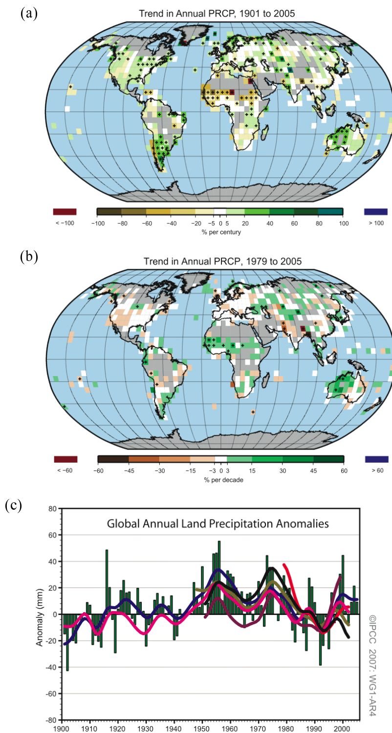
圖 3 (a)年平均降雨在 1901~2005 年期間的線性趨勢（單位： \% (100\text{yrs})^{-1} ）；(b)年平均降雨在 1979~2005 年期間的線性趨勢（單位： \% (10\text{yrs})^{-1} ）；(c)全球陸地平均降雨相較於 1961~1990 年之間平均值的變化。（摘自 IPCC 第四次評估報告，圖 TS.9）
