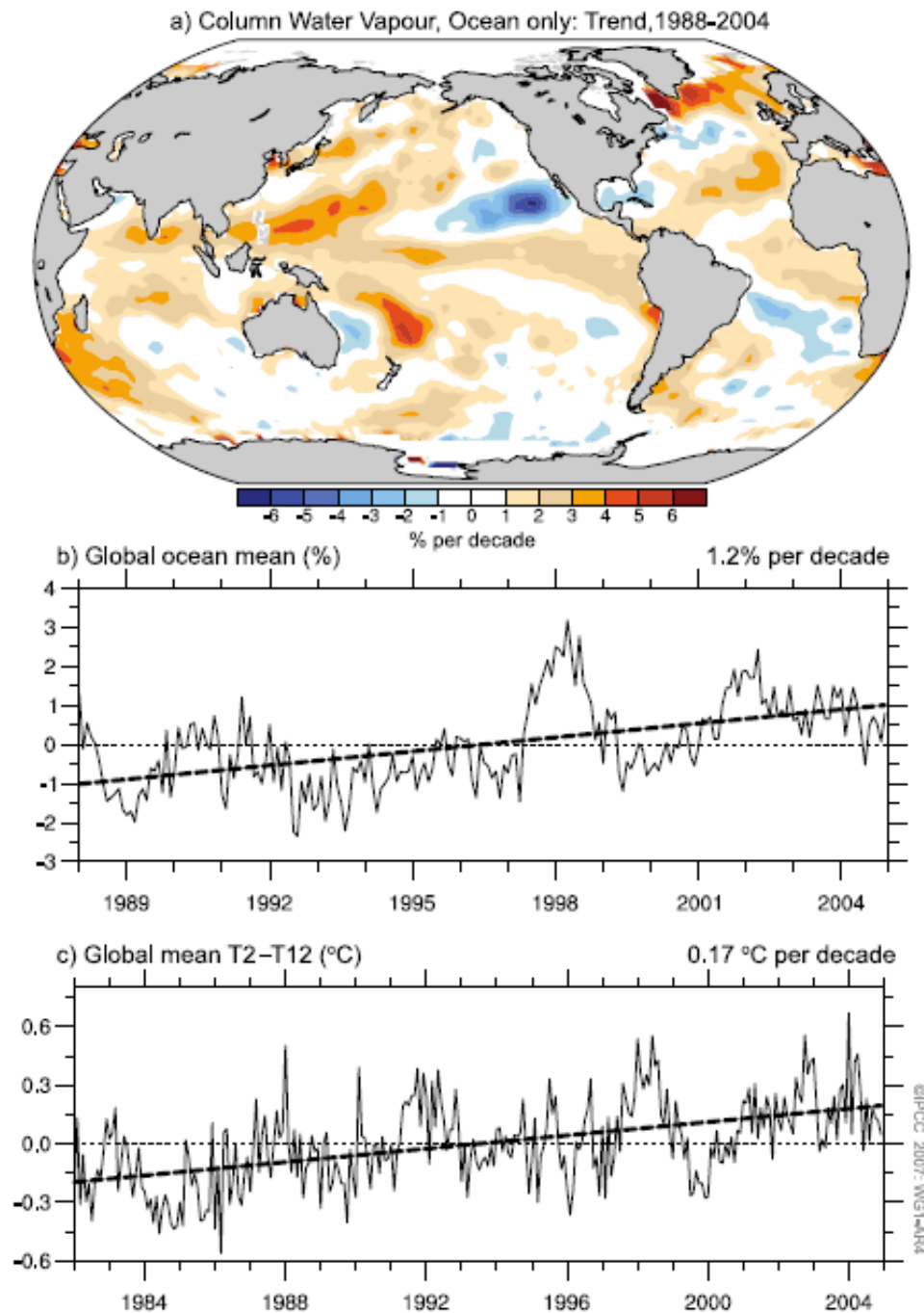
圖4 (a) 1988 年至 2004 年可降水量（總水氣含量）的線性趨勢( \% 10\text{yr}^{-1} )，(b)相對於此段時期全球海洋可降水量的逐月變化及線性趨勢，(c)相對於 1982 年至 2004 年之全球平均（80°N 至 80°S）的高對流層輻射亮溫（可代表水氣含量）的逐月變化(°C)，虛線表示亮溫的線性趨勢，以每十年多少°C 表示。（摘自 IPCC 第四次評估報告，圖 TS.8）
