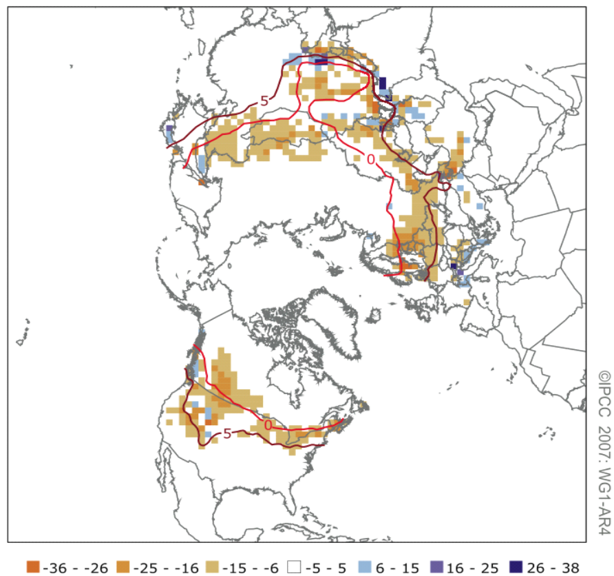
圖9 北半球冰雪覆蓋面積的變化和空間分佈。(摘自 IPCC 第四次評估報告，圖 TS.12)
