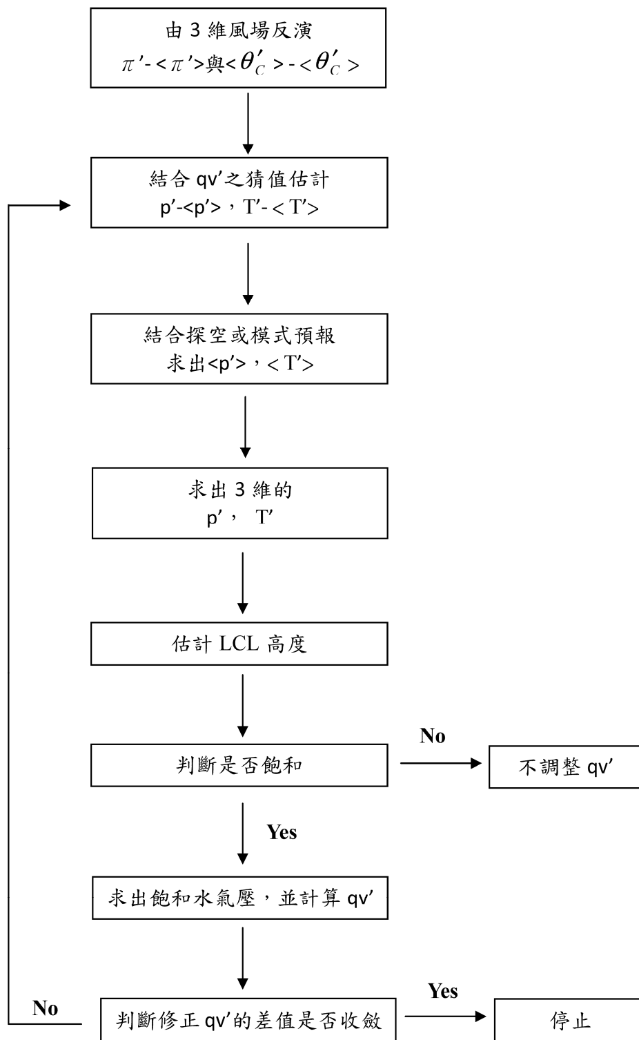
圖 1 調整水氣混合比擾動場( q'_v )的流程。
