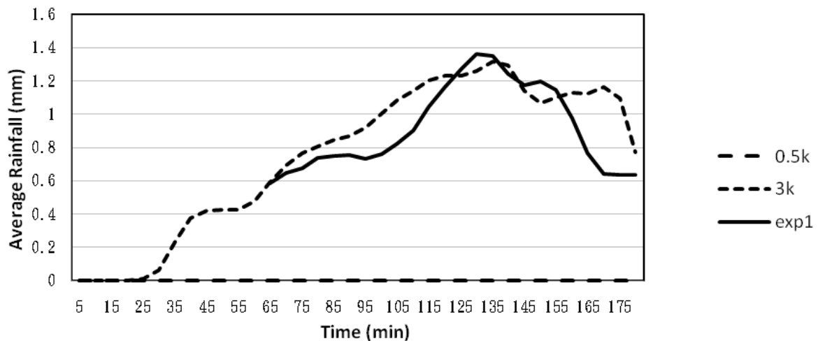
圖 5 實驗 1 與「natural run」於模擬區域內有降雨網格點上進行平均後，每五分鐘累積降雨量隨時間變化圖。長虛線為無同化實驗；短虛線為 natural run；實線為實驗 1 的結果。橫坐標為模式模擬的時間，資料同化發生在第 60 分鐘時。
