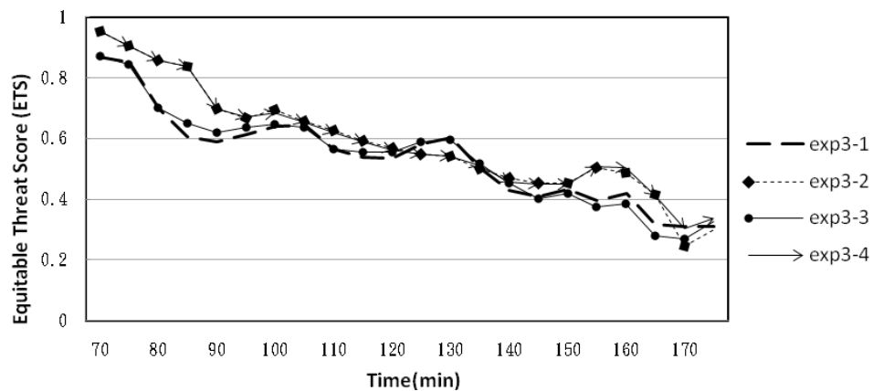
圖 9c 同圖 9a，但是為五分鐘累積降雨量 ETS 得分隨時間的變化圖。
