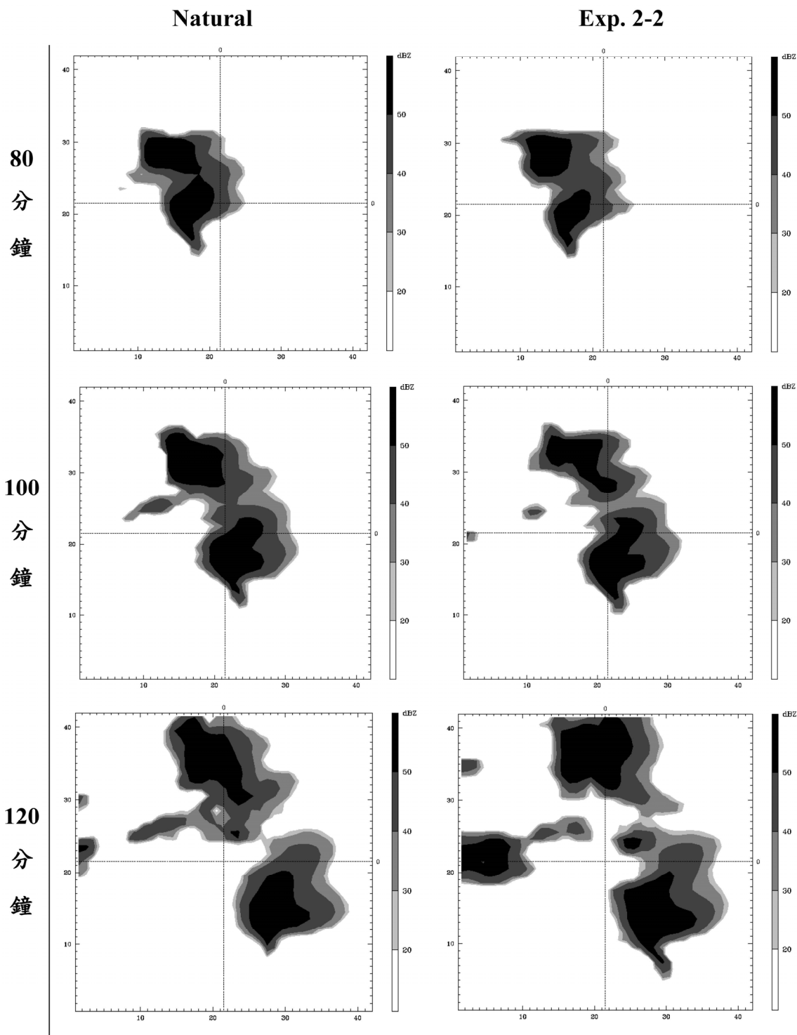
圖 7 Natural run (左圖)與實驗 2-2(右圖)在模擬時間第 80、100 及 120 分鐘時的回波場。
