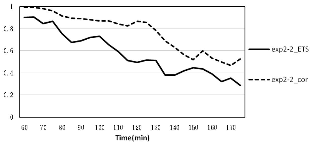
圖 8b 實驗 2-2 和「natural run」五分鐘累積降雨量相關性(虛線)、「ETS」得分(實線)隨時間變化圖。
