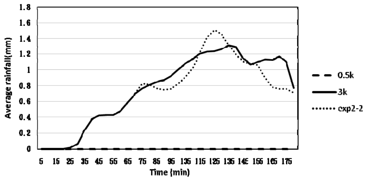
圖 8a 實驗 2-2(點線)、「natural run」(實線)於模擬區域內五分鐘累積降雨量隨時間變化圖。長虛線為無同化結果。
