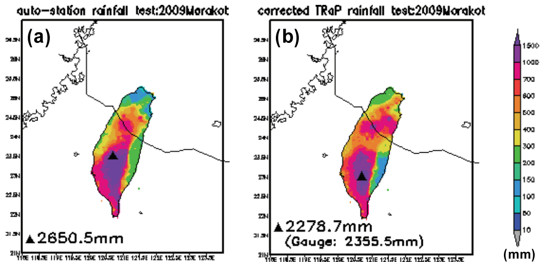
圖 4 (a)莫拉克颱風期間台灣地區測站之累積降雨，(b)考慮颱風強度變化、地形效應及季風共伴效應，改進 TraP 降雨模式所計算之累積降雨及其分布，圖中黑線為莫拉克颱風之移行軌跡（劉振榮、林唐煌、劉崇治提供）。
