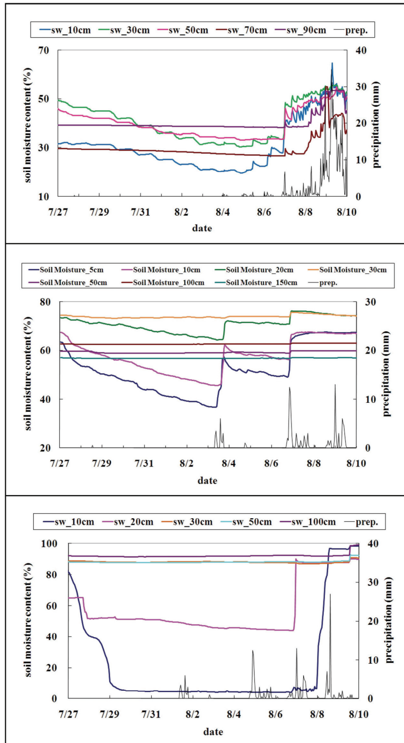
圖 11 2009 年 7 月 27 日~8 月 10 日於南投魚池鄉林試所蓮花池（上）、中央氣象局嘉義測站（中）以及颱風研究中心嘉義東石測站（下）不同深度的土壤含水率觀測值。
