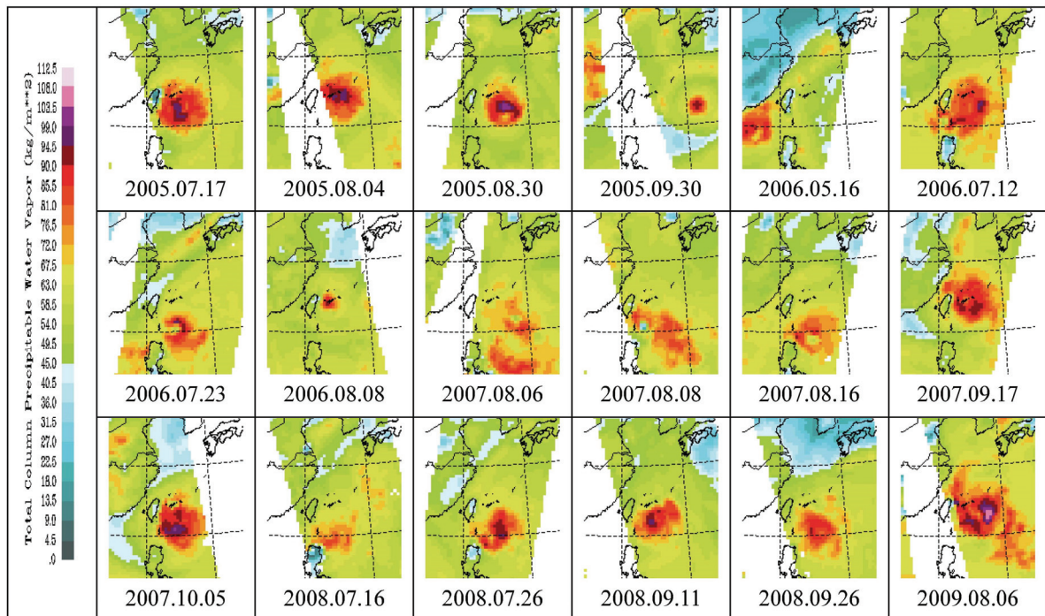
圖 1 2005~2009 年 18 個侵臺颱風個案衛星反演西北太平洋的可降水量，圖中的右下角(2009.08.06)個案即為莫拉克颱風（周鑑本、吳倩雯、齊祿祥、張拱祿、廖美慧等提供）。
