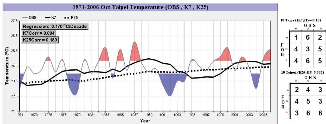
圖4 臺北測站10月觀測溫度、K值為7與K值為25之時間序列圖。圖中細實線為觀測值，粗實線是K值為7，粗點線是K值為25。左上角數字分別為觀測之迴歸趨勢值、觀測值與K=7之相關係數與觀測值與K=25之相關係數值。圖右分別為觀測值與K=7及觀測值與K=25之3分類表格，表中分別為:-:偏少類別，o:正常類別，+:偏多類別，HS代表3分類之預報技術得分。
