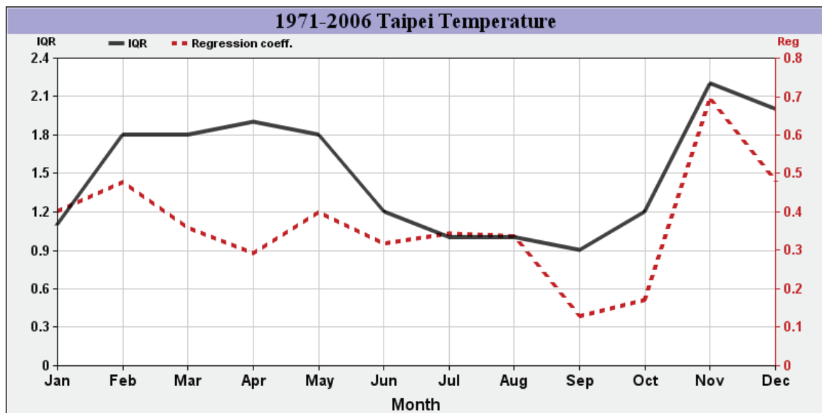
圖 7 臺北測站各月份之 IQR(實驗)與溫度趨勢值(點線)之時間序列圖。圖中 IQR 代表所有資料長度的第百分之 75 與第百分之 25 之間的差別，X 軸為月份，Y 軸分別為 IQR 值與迴歸趨勢值。
