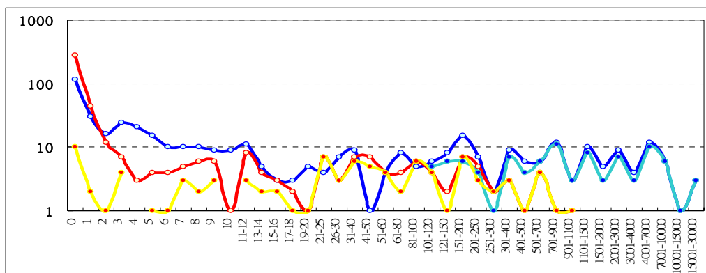
圖3 午後對流個案（青及黃色分別為 type01 及 type4）與全部 459 天（深藍及紅色分別為 type01 及 type4）之累積閃電次數—頻率。橫座標為累積閃電次數，縱座標為出現天數（對數座標）。
