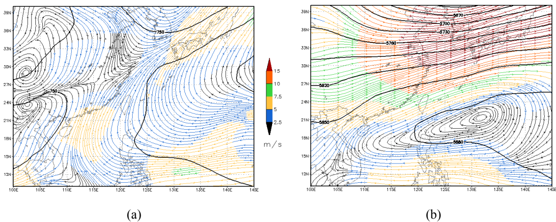
圖 6 五月份東區百分比值大於西區百分比值個案之合成 (a) 925 hPa 及 (b) 500 hPa 氣流線與等高線（間距 30 gpm）。各圖色階均為風速，單位為 ms^{-1} 。
