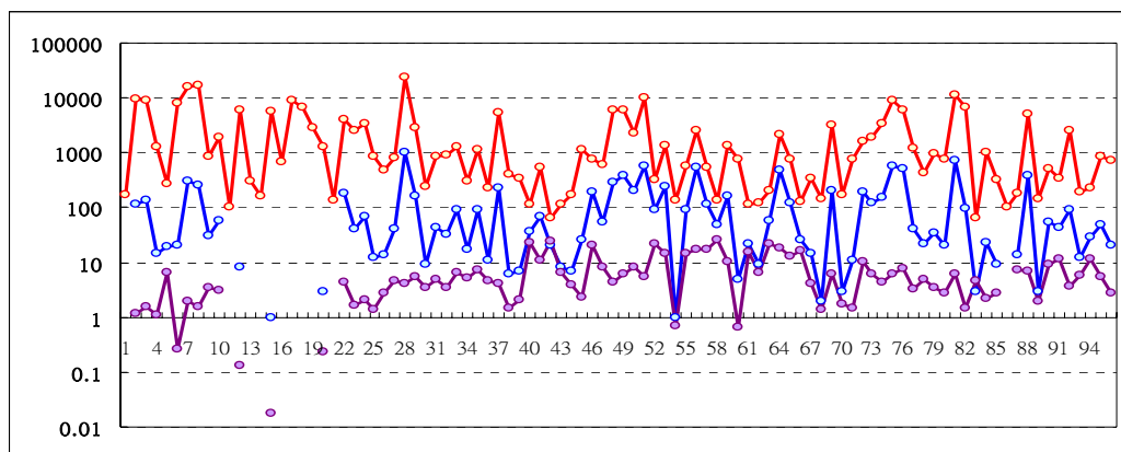
圖 4 午後對流個案的 type4、type014 及其比值 (%)（分別為深藍、紅及紫色）。橫座標為個案編號（表一），縱座標已取對數刻度，致部份個案資料落點因數據為 0 而無法相連。
