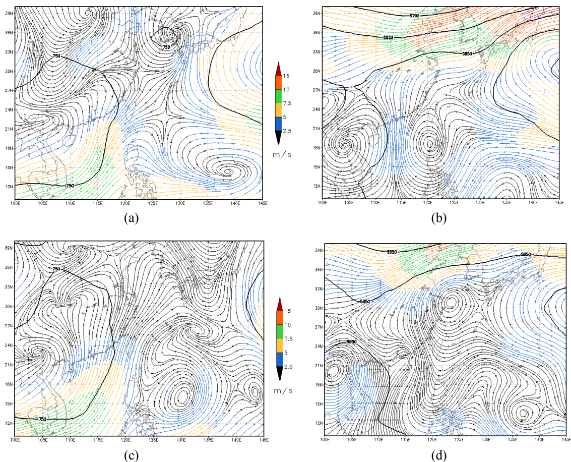
圖 10 同圖 8，但均為八月份。
