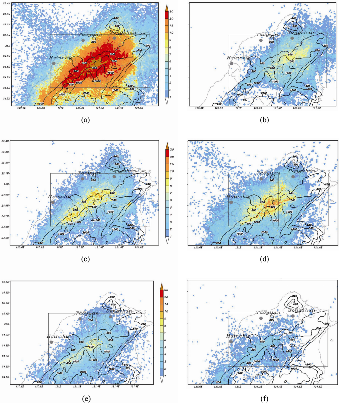
圖2 臺灣北部 (a) 五至九、(b) 五、(c) 六、(d) 七、(e) 八及 (f)九月份午後對流出現天數(色階)的時、空分布(不含一天以下)。各圖粗黑實線分別為海拔 200、500 及 1000 公尺高度,灰色框為本文所定義的北部地區。
