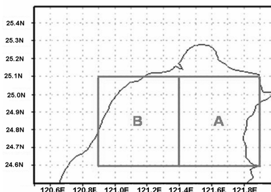
圖 1 個案選擇時所選取的分析範圍，及本文所定義的北部地區（紅色框）。東、西為分析各月份平均標準化閃電次數百分比值時所區分的區域。
