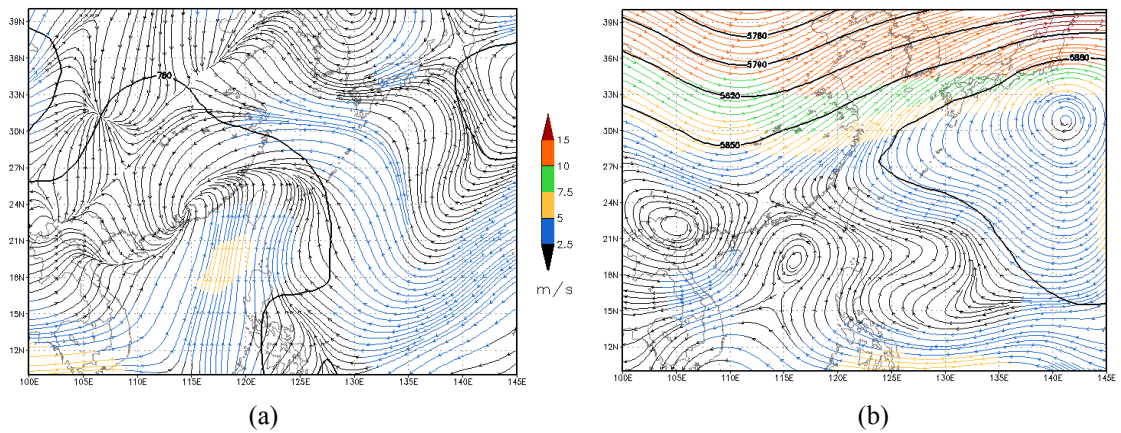
圖 7 九月份西區百分比值大於東區百分比值個案之合成 (a) 925 hPa 及 (b) 500hPa 氣流線與等高線 (間距 30 gpm)。各圖色階均為風速，單位為 ms^{-1} 。
