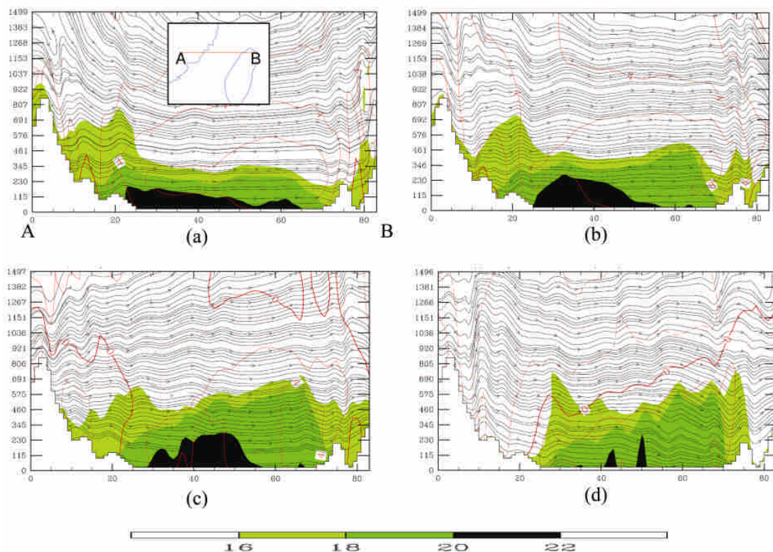
圖 13 通過五分山同一緯度切線之氣流場與水氣剖面。(a)3 日 18 UTC·(b)3 日 21 UTC·(c)4 日 00 UTC·(d)4 日 03 UTC，切線位置標示於(a)中，五分山位於最右側，各圖垂直軸為高度(m)，橫軸為格點數，每一點為 5 km，紅色等值線為風場南北分量(v)，間隔為 2\text{ ms}^{-1} ，負值為虛線，黑線則為東西風場分量(u)與垂直風場(w)的氣流線，顏色表示混合比( \text{g kg}^{-1} )，標示如圖。
