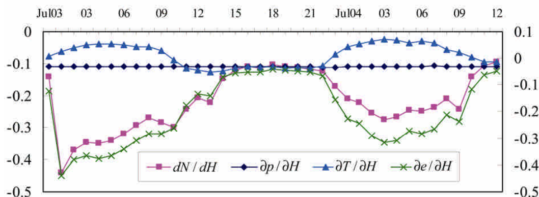
圖 10 五分之山之折射率、溫度、溼度與氣壓之垂直梯度時序圖，左側刻度為氣壓梯度 ( \partial p / \partial H , \text{hPa m}^{-1} )及折射率梯度( dN / dH , \text{N-Unit m}^{-1} )，右側則為溫度梯度 ( \partial T / \partial H , ^{\circ}\text{C m}^{-1} )及水氣壓梯度( \partial e / \partial H , \text{hPa m}^{-1} )
