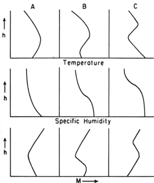
圖 3 產生大氣導管的典型環境特徵氣象因子高度分布圖，垂直軸為高度，上圖為溫度、中間為水氣，下圖則為修正折射率。（摘自 Battan, 1973）
