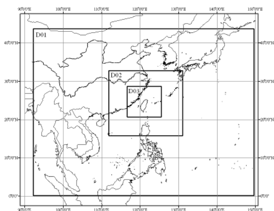
圖 6 模式三重網格設計，採用橫麥卡脫投影，以各網格範圍經緯度座標繪製而成。
