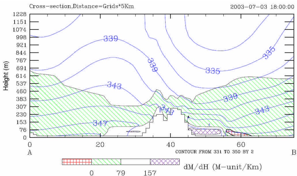
圖 4 2003 年 7 月 3 日 18 UTC 全球分析場繪製台灣北部大氣折射效應，折射效應閾值如色標所示，次折射為 dM/dh > 157 \text{ M km}^{-1} 、正常為 79 < dM/dh \leq 157 \text{ M km}^{-1} 、超折射為 0 < dM/dh \leq 79 \text{ M km}^{-1} 及陷捕為 dM/dh \leq 0 \text{ M km}^{-1} ，藍色線為相當位溫(K)，間隔為 2 K。切線位置如圖所示，垂直軸為高度(m)，橫軸為網格點數，每一格點 5 km，圖中空白無資料部分為地形，五分山雷達站相對位置為紅色箭頭所示。
