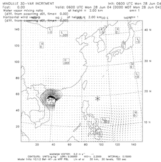
圖 11 同圖 10 但為使用個案 MGR 減去個案 MG 的離地表二公里處所得的水氣增量( g\ kg^{-1} )在 00h 的增量圖。
