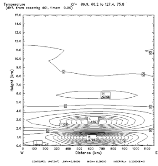
圖 4 (a)個案 HGR 減去個案 HG 的離地表 1 公里處所得的溫度增量( ), 星號(*)為當時颱風中心, 十字(+)為兩個掩星事件點。(b)以台灣東方洋面上的掩星事件點(緯度 22.25; 經度 134.59) 為中心的東西向高度剖面圖。
