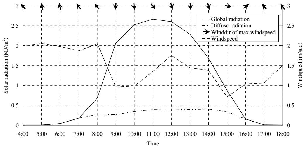
圖 6 2007/12/02 分析個案當日全天空輻射量、漫射光輻射量、風速與風向時序變化。
