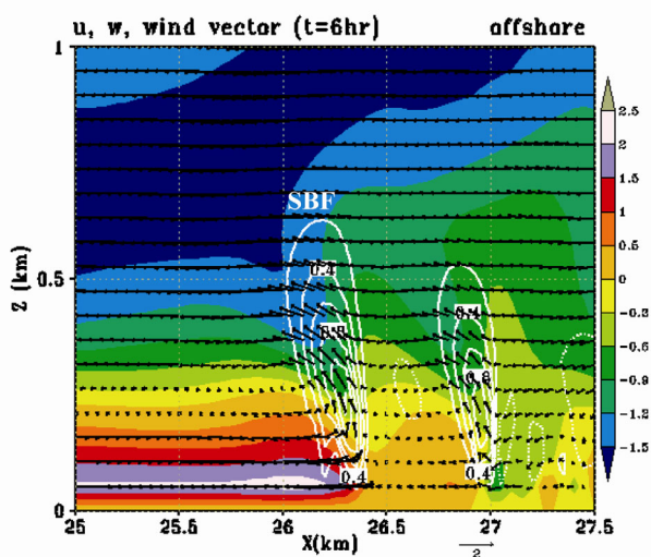
圖 12 同圖 4，但為個案 B2，25 至 27.5 km。
