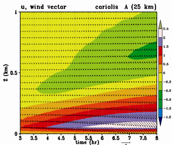
圖 5 個案 A 在 A 點（圖 1 第 25 km 處）水平風場 u（色階部分）和 u、v 合成風場（風標部分）綜合時間序列圖。
