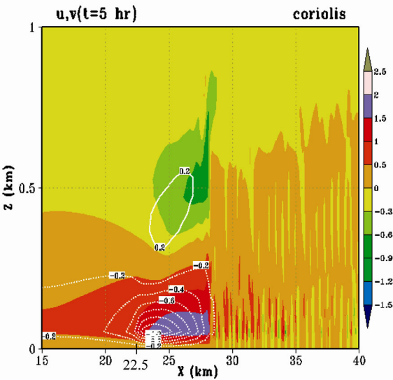
圖 2 個案 A 積分 5 小時後(11 時)，15 至 40 km 水平風場 u (色階部分，正值代表西風、負值代表東風)和 v (實線代表南風、虛線代表北風)的綜合結果，等值線間距均為 0.2 \text{ m s}^{-1} 。
