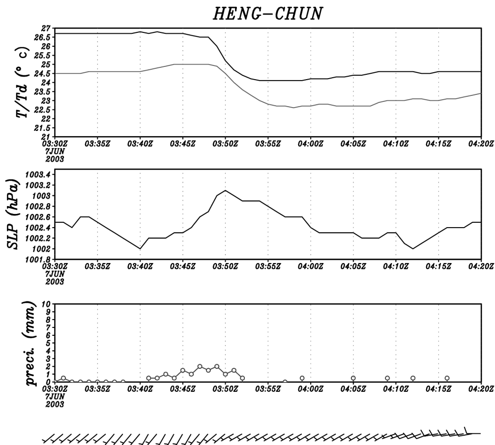
圖 8 2003 年 6 月 7 日 0330 至 0420 UTC 恆春測站每分鐘溫度、露點、海平面氣壓與降水等氣象因子時間序列圖。(資料來源：中央氣象局)
