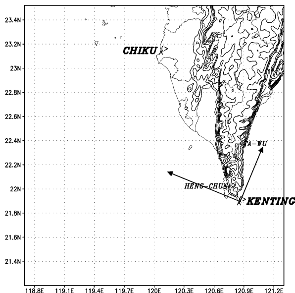
圖 2 台灣南部都卜勒氣象雷達網區域圖，包含七股（Chiku）、墾丁（Kenting）等兩座雷達，其中墾丁雷達位置上兩線交角處為扇形空白（sector blanking）區。
