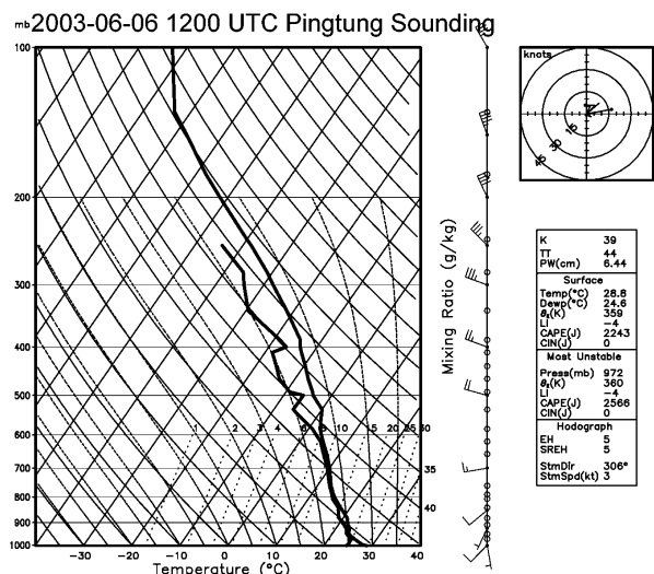
圖 4 2003 年 6 月 6 日 1200 UTC 屏東探空測站之斜溫圖。
