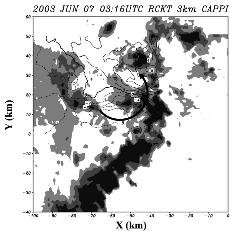
圖 11 同圖 10.，但時間為 2003 年 6 月 7 日 0316 UTC，粗實線為圖 9b 之垂直剖面位置。
