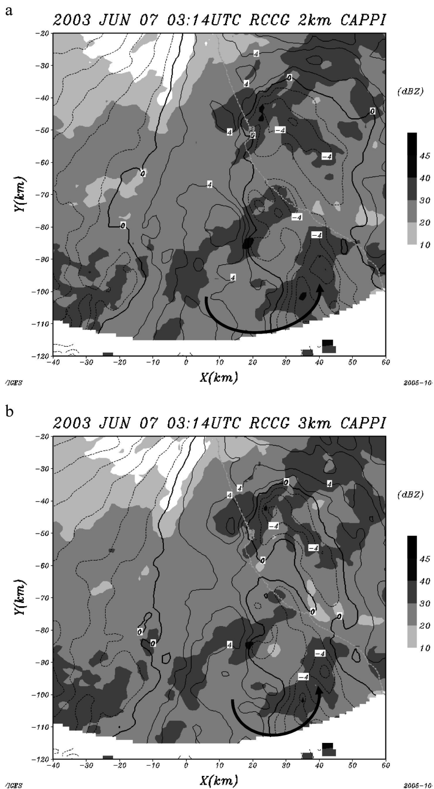
圖 13 同圖 12，但時間為 2003 年 6 月 7 日 0314 UTC。
