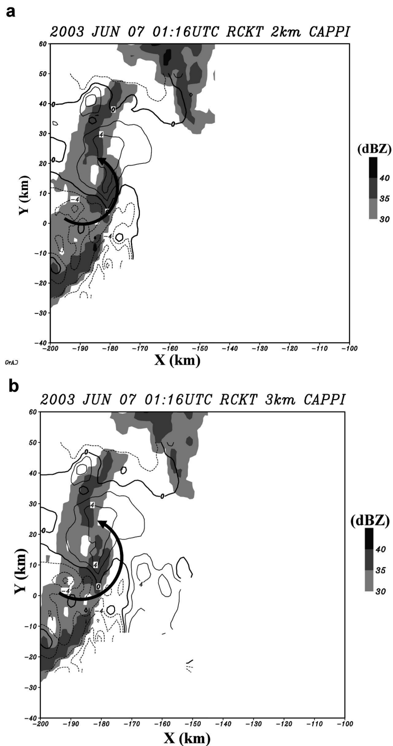
圖 10 2003 年 6 月 7 日 0116 UTC 墾丁雷達等高面平面位置顯示圖。(a) 高度 2 公里，(b) 高度 3 公里。等值線為濾除系統移速後之都卜勒風場（間距為 2 m/s），陰影區為降水回波（dBZ）。箭矢曲線所指之處為都卜勒風場偶極區，代表渦旋的位置。X 與 Y 軸分別為相對於雷達位置（0, 0）之東西向與南北向的距離（km）。
