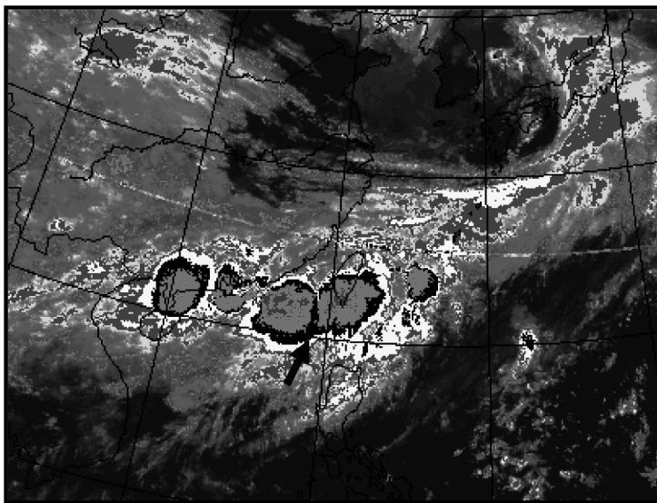
圖 5 2003 年 6 月 7 日 0000 UTC 東亞地區 GOES-9 紅外線加強色階衛星雲圖，圖中粗黑箭頭標示亮度溫度較高的帶狀區。
