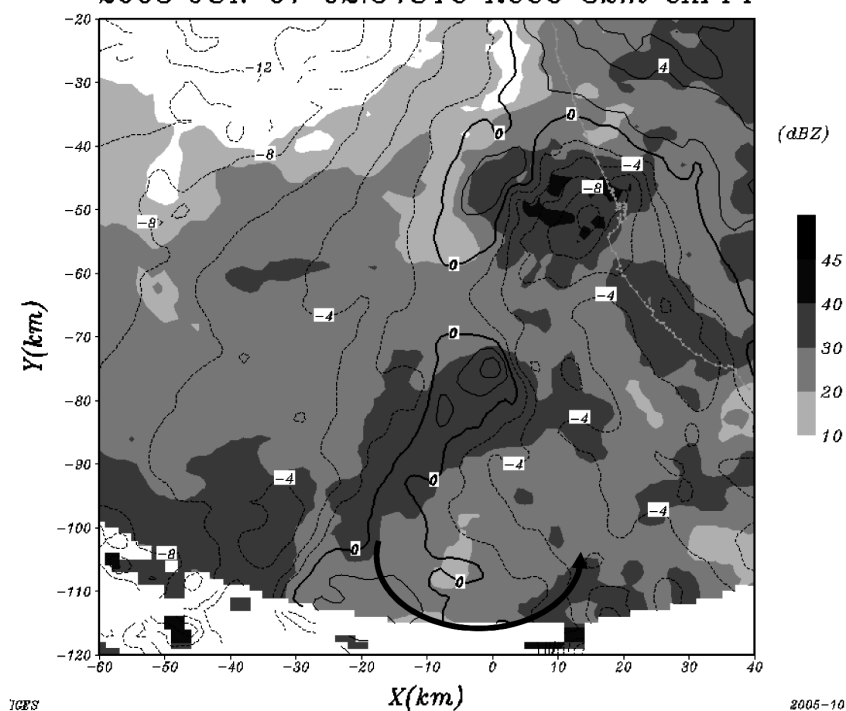
圖 12 2003 年 6 月 7 日 0254 UTC 七股雷達的等高面平面位置顯示圖。(a) 高度 2 公里，(b) 高度 3 公里。等值線為都卜勒風場強度（間距為 2 m/s），陰影區為降水回波（dBZ）。箭矢曲線所指之處為都卜勒風場偶極區，代表渦旋的位置。X 與 Y 軸分別為相對於雷達位置（0, 0）之東西向與南北向的距離（km）。
