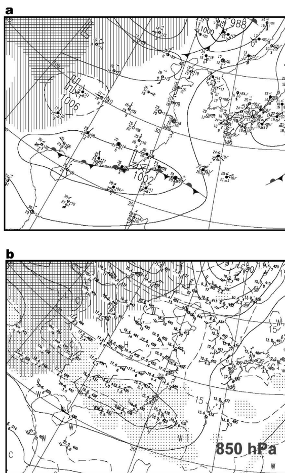
圖 3 2003 年 6 月 7 日 0000 UTC 天氣圖。(a) 地面分析圖, (b) 850 hPa 高空分析圖。(來源: 日本氣象廳)
