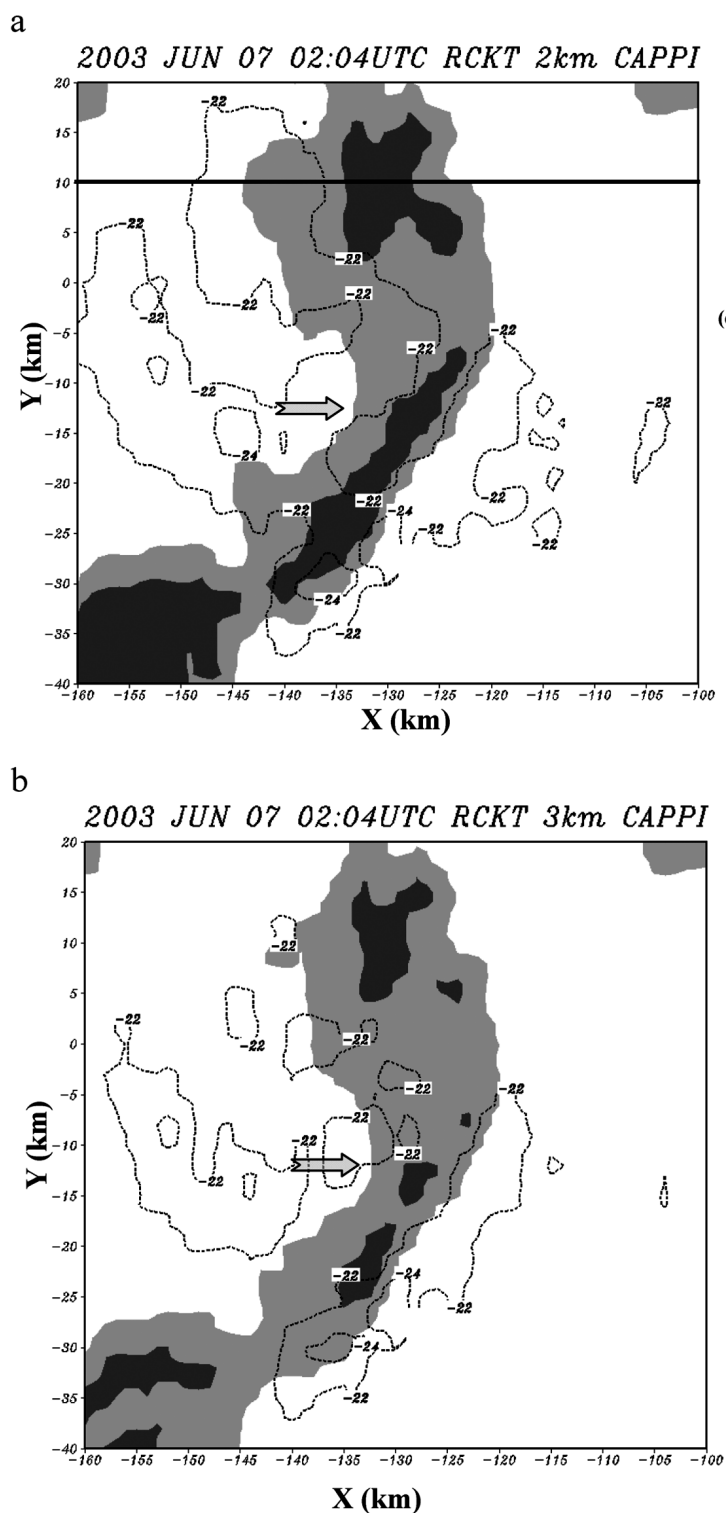
圖 7 2003 年 6 月 7 日 02040 UTC 墾丁雷達的等高面平面位置顯示圖。(a) 高度 2 公里，(b) 高度 3 公里。等值實線為強度 30 dBZ 之降水回波，虛線為 -22 \text{ ms}^{-1} 與 -24 \text{ ms}^{-1} 之都卜勒風場，陰影區分別為強度大於 30 與 40 dBZ 之降水回波區。箭矢所指之處為後方入流凹區 (rear-inflow notch)，粗實線為垂直剖面位置 (圖 9a)。
