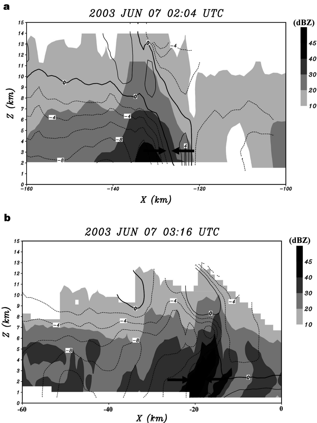
圖 9 2003 年 6 月 7 日墾丁雷達垂直剖面圖，(a) 0204 UTC，(b) 0316 UTC。箭號代表徑向風輻合區，剖面位置如圖 7a 與圖 11a 之粗實線所示。X 軸為相對於雷達位置 (0, 0) 之東西向距離 (km)，Z 軸為高度，等值線為濾除系統移速後之都卜勒風場 (間距為 2 m/s)，陰影區為降水回波 (dBZ)。
