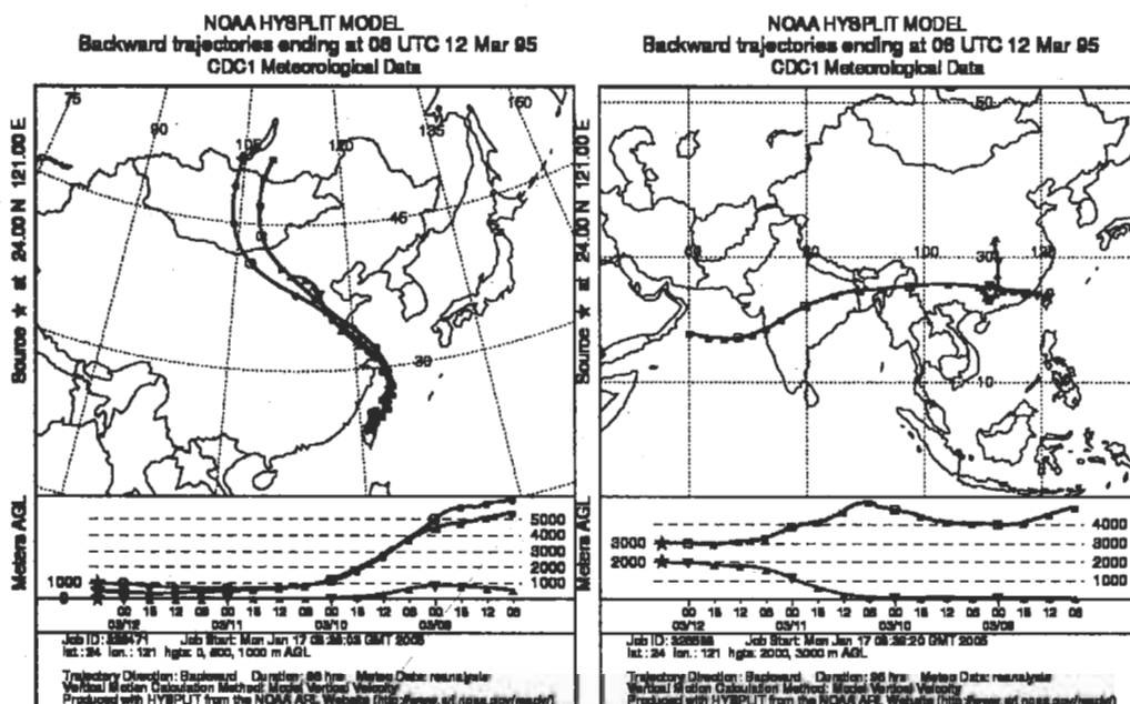
圖4 1995 年 3 月 12 日由台灣北部地區往後推估三日之軌跡線分析，後推起始點高度採用地面、500 和 1000 公尺(左圖)，以及 2000 和 3000 公尺(右圖)。軌跡線分析採用 NOAA/HYSPLIT 軌跡線模式，該模式採用 MM5 輸出三維風場推導軌跡線。
