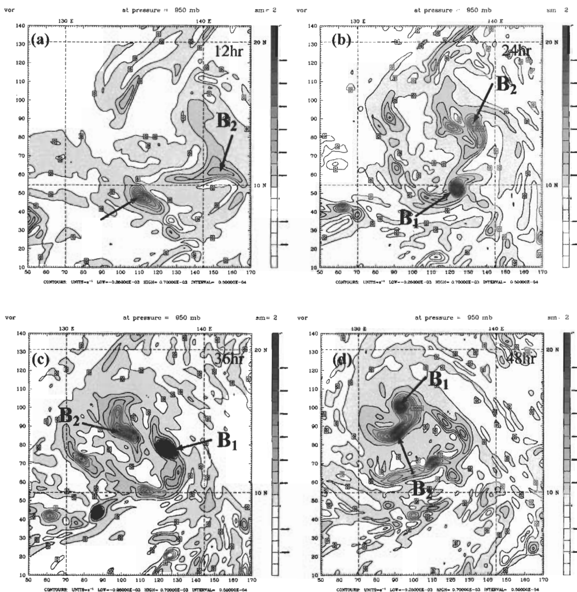
圖 11 模式所模擬之歐珀颱風(1997)個案的 950hPa 相對渦度場，等值線間距為 5.0 \times 10^{-5} \text{s}^{-1} ，圖中右上角標示模擬積分時間， B_1 和 B_2 分別標示兩渦旋之渦度中心。
