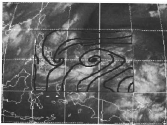
圖 16 1997 年 7 月 17 日 0000UTC 之紅外線衛星雲圖和 ECMWF 資料之 850hPa 流場，圖中央右方之環流為羅絲颱風(Rosie, 1997)之初始擾動。
