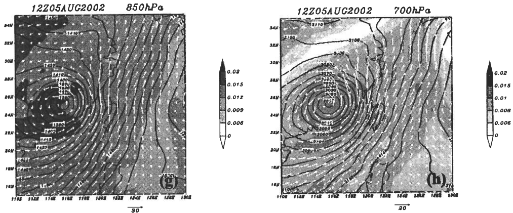
圖 9 2002 年八月五日 0000 UTC(a)1000 hPa、(b)925 hPa、(c)850 hPa、(d)700 hPa 及 1200 UTC(e)1000 hPa、(f)925 hPa、(g)850 hPa、(h)700 hPa 綜觀天氣圖。陰影區為混合比，單位為 g\ kg^{-1} ，間距如各圖右色階；白色箭頭為風向量，風速大小如各圖下方尺標，單位為 ms^{-1} ；黑色實線為等重力位高度，間距為 10。
