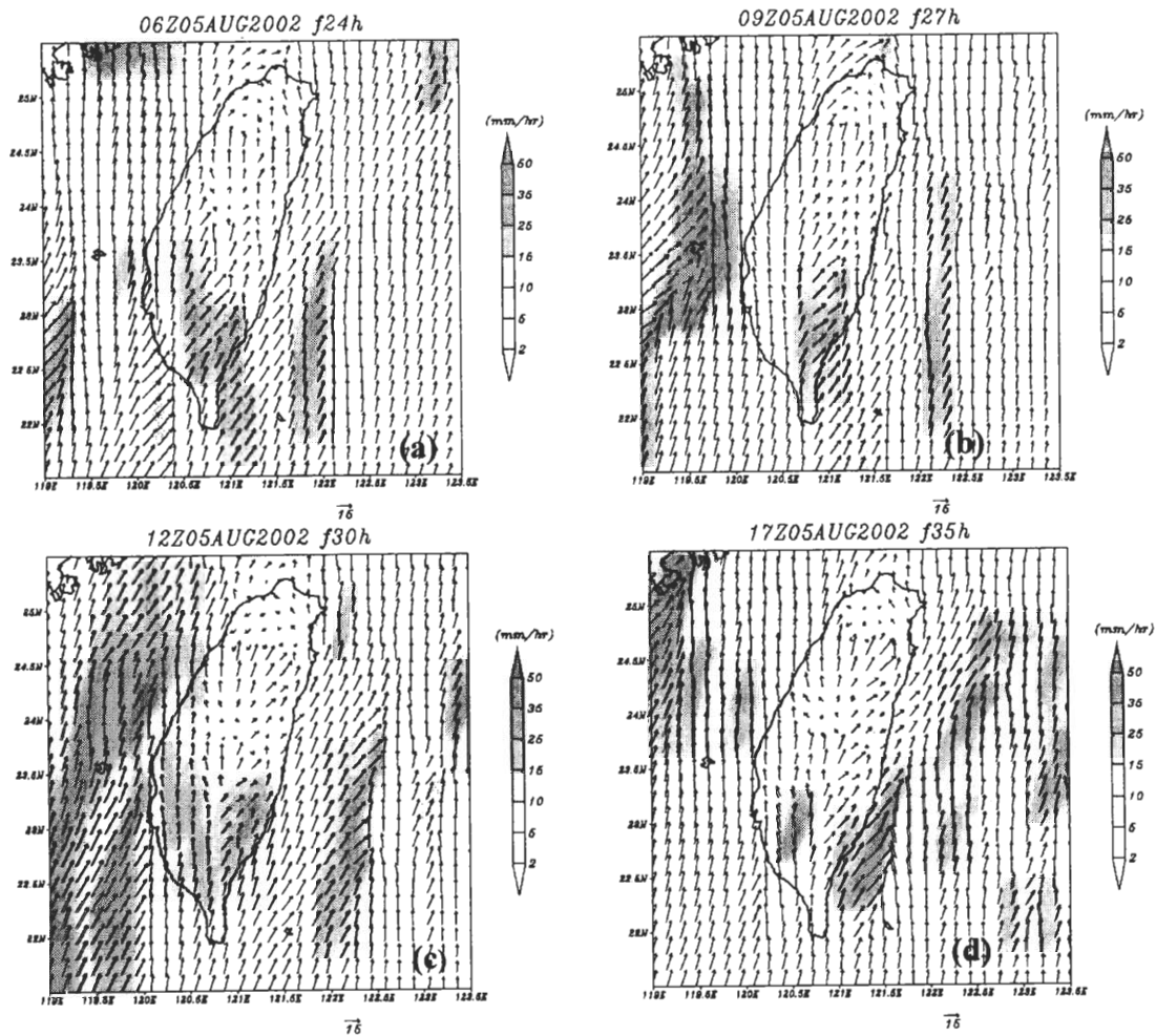
圖 13 MSM4 模擬之距地表 10 公尺高度風場與時雨量；圖(a)為模擬第二十四小時(八月五日 0600 UTC)、(b)為模擬第二十七小時(八月五日 0900 UTC)、(c)為第三十小時(八月五日 1200 UTC)及(d)為模擬第三十五小時(八月五日 1700 UTC)之結果。圖中陰影區為時雨量，單位為 mm\ hr^{-1} ，間距參考各圖右色階；箭號為 10 公尺高度風場，單位為 ms^{-1} ，風速大小參考圖右下尺標
