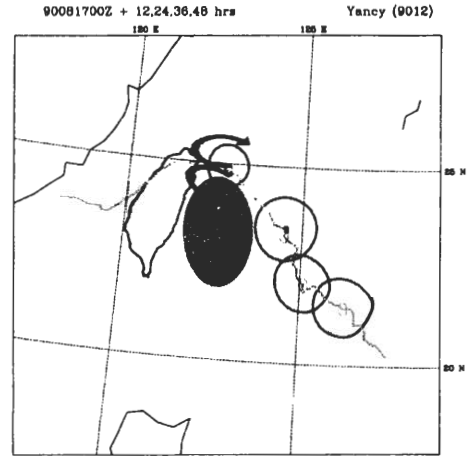
圖 24 Yancy 路徑呈現大角度北偏後，又轉回西北加速，並以偏西之角度登陸台灣北端的概念圖，圖中陰影區有顯著水平正角動量通量平流，箭號代表台灣地形破壞颱風結構所引發之通風氣流。
