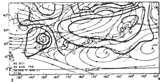
圖二 一九六一年八月卅日地面等壓線(斷線)與三萬英尺氣流線(實線)(Sadler 1963)
