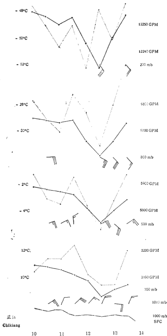
圖十七 六十四年八月十日及十四日芷江時間垂直剖面圖 (虛線表溫線；實線高度)
