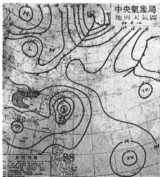
圖六 六十四年八月十二日八時地面圖 Fig. 6 Surface chart for 00Z August 12, 1975.
