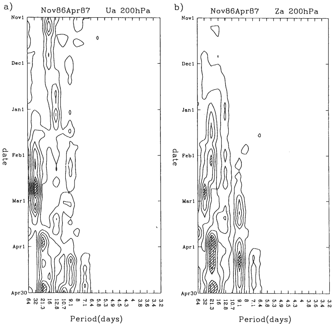
圖 7 200 百帕緯向風速及重力位高度距平時間序列之移動波譜。緯向風速之等值間距為 200 m^2/s^2 、陰影區域為 \geq 800 m^2/s^2 而重力位高度之等值間距為 10^6 m^2 、陰影區域為 \geq 5 \times 10^6 m^2 。
