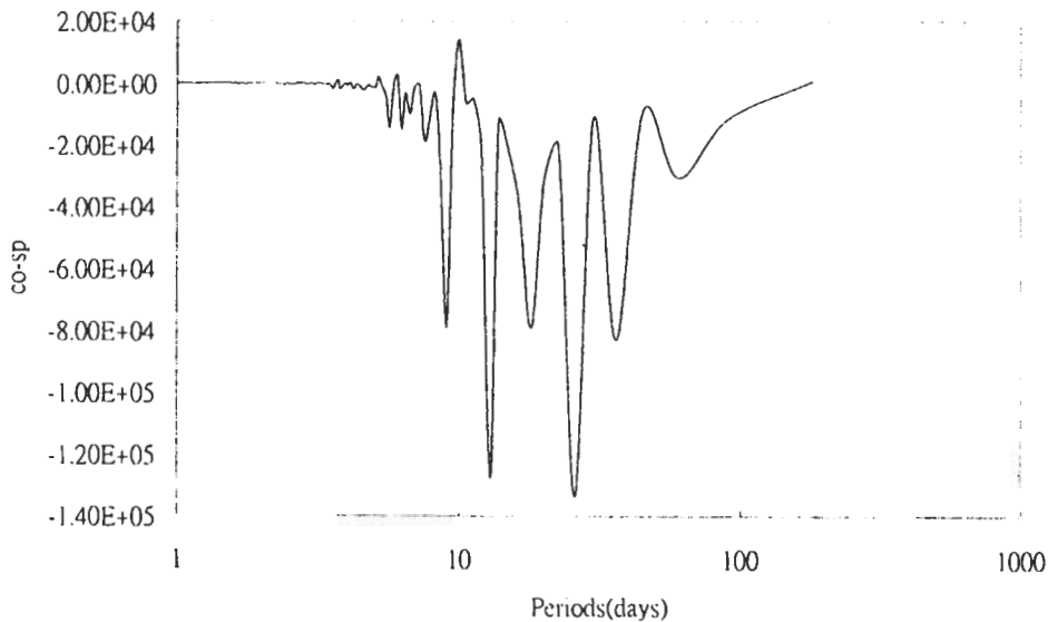
圖 8 200 百帕緯向風速及重力位高度距平時間序列之同相波譜。
