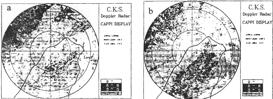
圖 2 1991-1996 年 5-6 月(a)鋒面型與(b)非鋒面型午後初生 ≥ 15 dBZ 對流之頻率分布。雷達掃描半徑內圈、中圈及外圈分別為 50 公里、100 公里及 120 公里。
