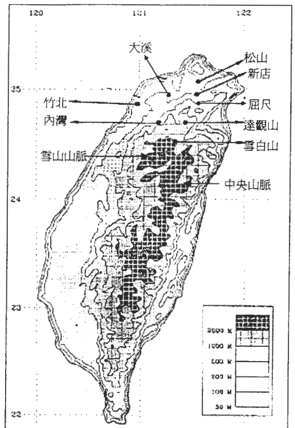
圖 1 1 公里網格間距地形高度，經 5 公里 \times 5 公里勻滑之地形等高線與各地回波分析所在位置。
