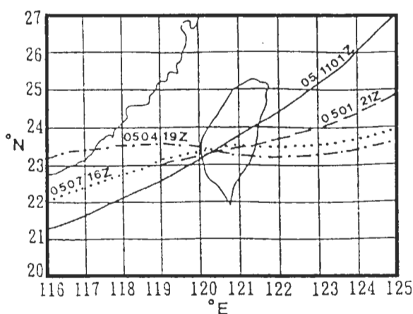
圖3 1996年5~6月移經台灣中南部之四道鋒面於 t=0 時所在位置。鋒面上6位數字每2位分別為月、日及國際時。
