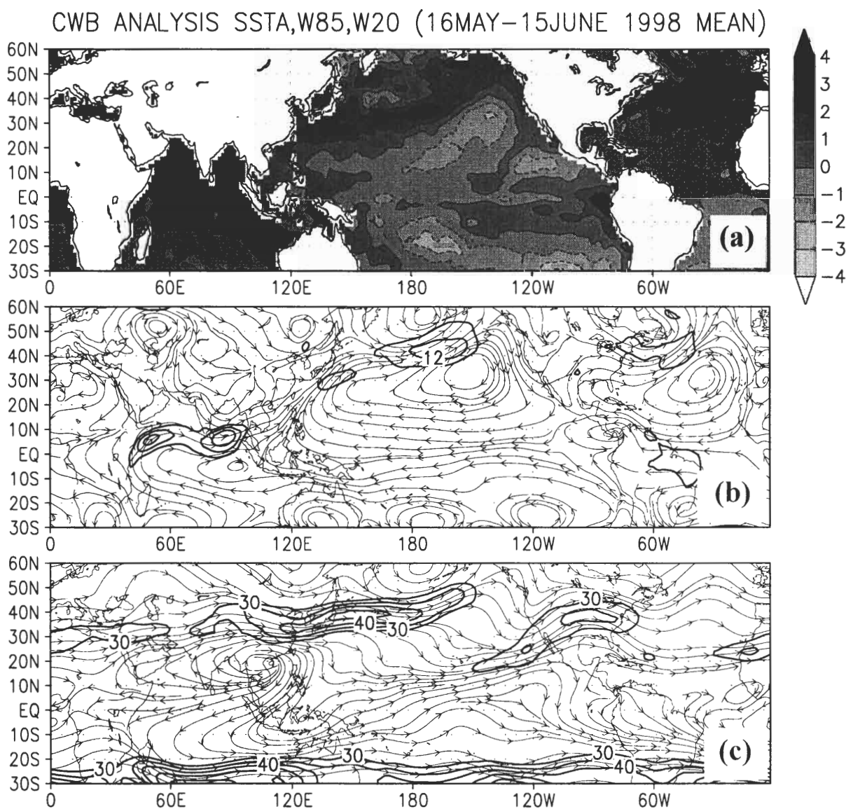
圖 3 實驗期間平均之海溫距平及水平環流分析圖。
