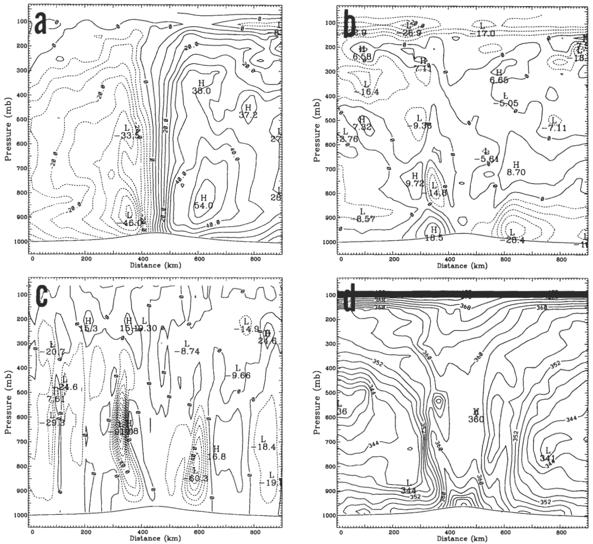
圖 5 實驗 KF00 積分 24 小時時通過颱風中心之東西向垂直剖面圖；分別為南北向和東西向風速 (a 和 b，等值線間距 5 m/sec)、垂直速度 (c，等值線間距 10 \mu bar/s) 及相當位溫 (d，等值線間距 2° K)。
