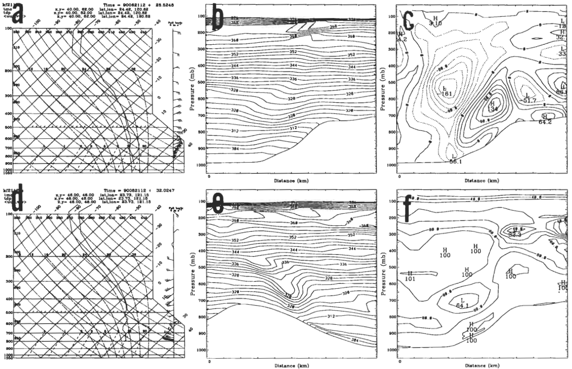
圖 13 圖 12 中 A 點和 B 點之濕溫垂直分佈斜溫圖 (a 和 d)，通過 A 點之位溫 (b，等值線間距 2° K)、垂直速度 (c，等值線間距 20 μ bar/s) 和相對濕度 (f，等值線間距 10%) 垂直剖面圖及通過 B 點之位溫垂直剖面圖 (e)；剖面位置如圖 12 所示。
