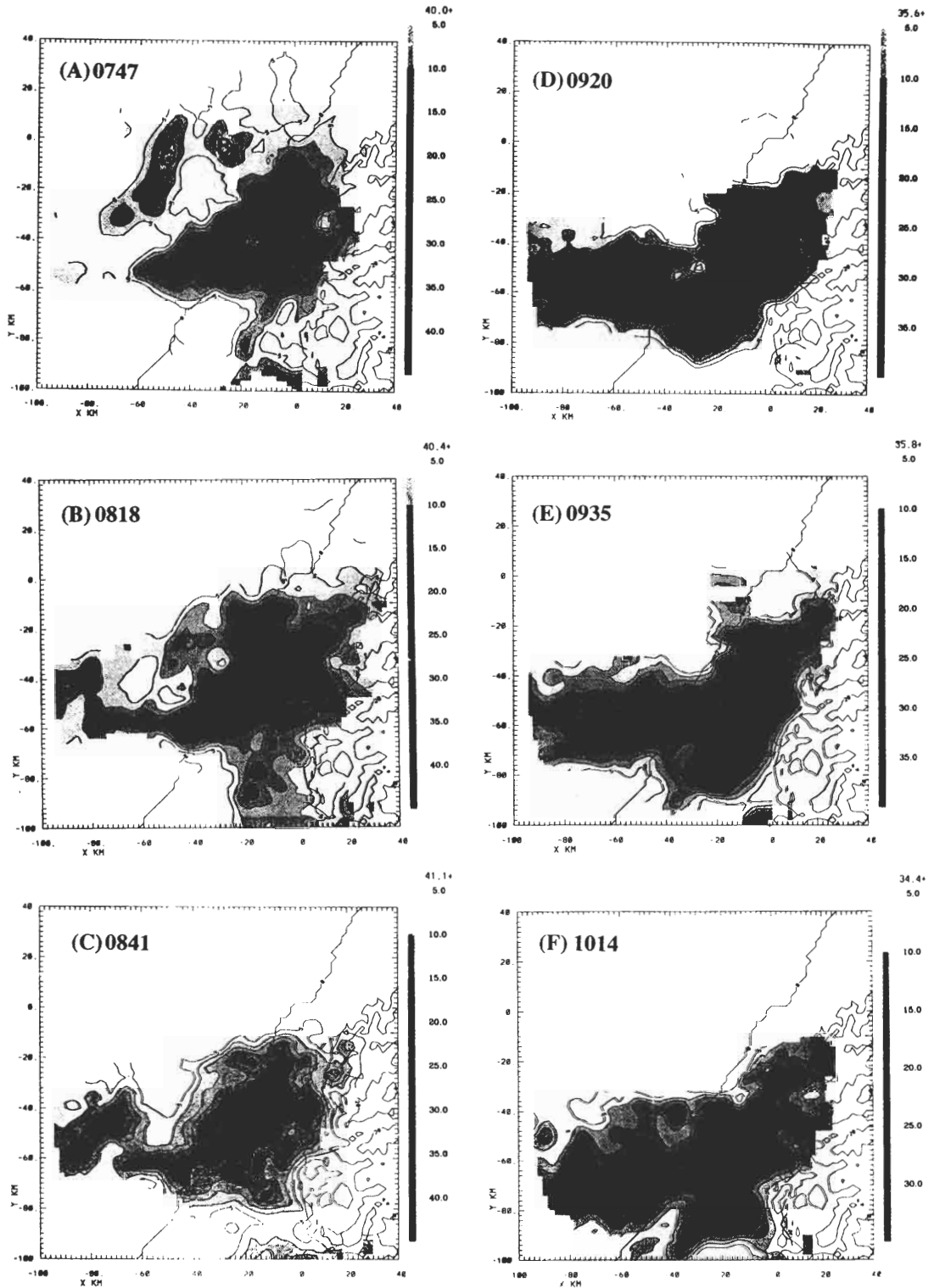
圖 4 TOGA 雷達在 1987 年 6 月 25 日 0747LST 至 1014LST 所觀測平均每隔 7 分鐘於 1km 高度的回波圖 (等值線間隔為 5dBZ) (地形等高線第一條線為 0m, 間隔為 500m)。(A)0747~0754, (B)0818~0825, (C)0841~0849, (D)0920~0927, (E)0935~0943, (F)1014~1022。
