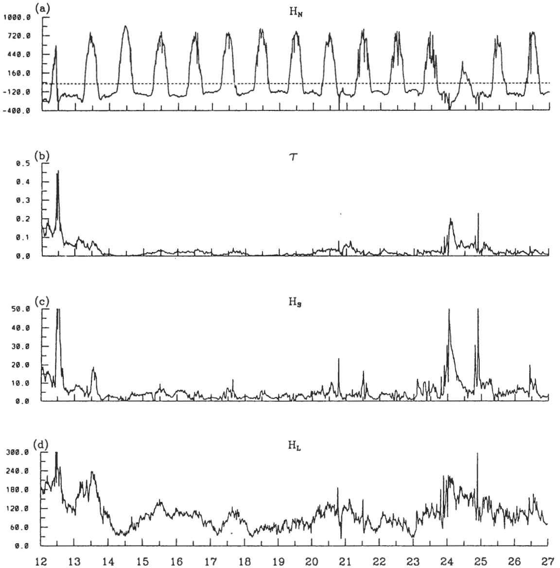
圖3 同圖2，但為海氣界面各種紊流通量。(a)海面淨熱通量( \text{W}/\text{m}^2 )，(b)風應力( \text{N}/\text{m}^2 )，(c)可感熱通量( \text{W}/\text{m}^2 )，(d)潛熱通量( \text{W}/\text{m}^2 )。
