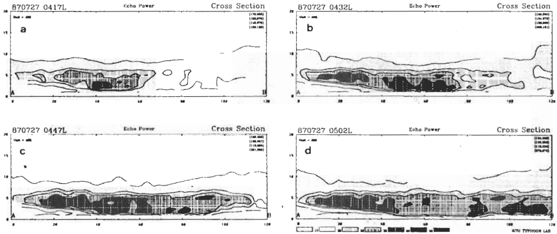
圖 19 亞力士颱風伴隨雨帶垂直剖面圖,垂直剖面所切之位置以圖 17 之粗實線表示。時間為(a)0417L (b)0432L (c)0447L和(d)0502L。
