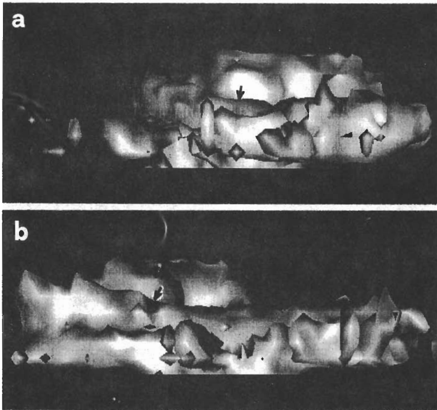
圖 20 1987年7月27日0502L,CAA雷達的降水回波資料,以AVS軟體顯示的立體等值面。分別為自(a)西方和(b)西北方平視。
