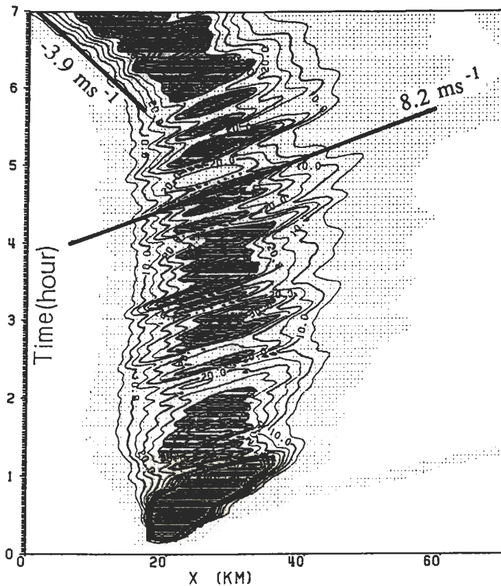
圖 31 三維颶線數值模擬結果，平行颶線方向之地面降水強度隨時間變化圖，陰影區表 30\text{mmh}^{-1} 以上，積分 5 小時開始在颶線後方加以面復迴流之外力，颶線向右傳播速度增加 3.9\text{m}^{-1} ，降水強度劇增 (Chang, 1991b)。
