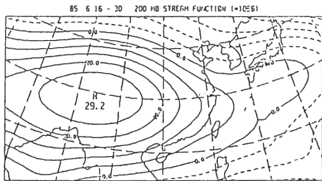
圖 6c 1985 年 5、6 月期間 15 天平均之 200mb 流函數場 ( \times 10^6 ，間距 5 \times 10^6 )
