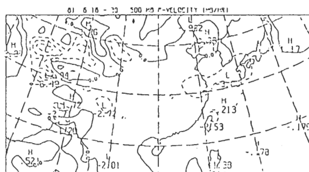
圖 1e 1981 年 5、6 月期間 15 天平均之 500mb 垂直速度場 (單位 mb/hr, 間距 2mb/hr)
