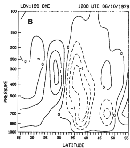
圖15 沿東經120度垂直速度之南北向垂直剖面，實線為上升速度，虛線為下降速度，等值線間距為 0.5 \times 10^{-3} hPa s^{-1} 。a) 1979年5月27日0000 UTC、b) 1979年6月10日1200 UTC。
