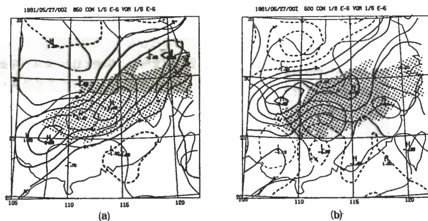
圖5 輻合（細——）、輻散（細---）每 2 \times 10^{-5} \text{ S}^{-1} 為間隔以及正渦度（粗——）、負渦度（粗---）每 2 \times 10^{-5} \text{ S}^{-1} 為間隔，雲圖位置（陰影區）。1981/05/27/00 Z：(a)為850 mb；(b)為500 mb。
