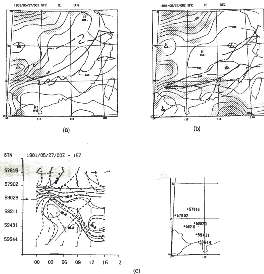
圖7 地面相當位溫 ( \theta_e ) 分佈 (細——) 每 5^\circ\text{K} 為間格。地面鋒面位置 (粗——), 雲團範圍 (粗---), |\nabla_H \theta_e| \geq 4^\circ\text{K}/100\text{Km} 區域 (陰影區)。1981/05/27: (a) 為 00Z; (b) 為 06Z; (c) 南北剖面時間序列圖及測站相對位置分佈: 相當位溫等值線 (細——) 每 5^\circ\text{K} 為間隔、溫度等值線 (粗——) 每 2^\circ\text{C} 為間隔水汽等值線 (細----) 每 2\text{g/Kg} 為間隔。箭號表示對流雲系出現的位置, 時間軸上之粗實線為雲系出現的時間。
