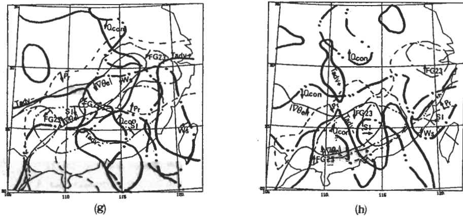
圖 15 七項分析因子交集區及其新生雲系位置分佈。FG 23 = 20^{\circ}\text{K}/1000\text{Km}/\text{DAY} 等值線 (細---), |\nabla_{\theta} \theta| = 4^{\circ}\text{K}/100\text{Km} 等值線 (細——), SI = 300 等值線 (細---), Pr = 60\text{mm} 等值線 (細----), Ws 700 = 4 \times 10^{-3} \text{S}^{-1} 等值線 (粗---), Tadv = 0 等值線 (粗——), Qcon = 0 等值線 (粗----), 箭號的指向為所要之區域。(a) 1981/05/27/00 Z, 對流雲系之時間為 06 Z; (b) 1983/06/16/00 Z, 對流雲系之時間為 09 Z; (c) 1984/05/31/00 Z, 對流雲系之時間為 06 Z; (d) 1987/05/15/12 Z, 對流雲系之時間為 15 Z; (e) 1986/05/20/12 Z; (f) 1986/06/04/00 Z; (g) 1984/06/14/12 Z; (h) 1984/06/16/15/00 Z。
