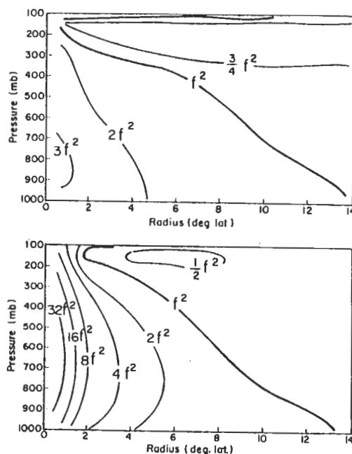
圖 19 TC 在積雲簇（上圖）和 TS（下圖，最大風速 43 kts）之慣性穩定度 ( I ) 平方值，（以 f 表示），上圖中心緯度為 11^\circ\text{N} ，下圖為 14^\circ\text{N} 。
