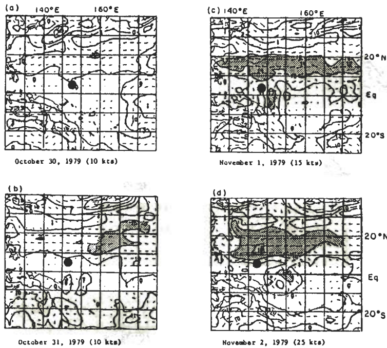
圖14 西北太平洋STY Vera 生成前之大範圍環流型式。黑點表系統中心位置，陰影區表風速大於10 kts。
