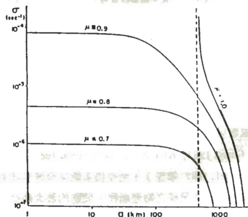
圖1 熱帶氣旋成長率( \sigma )和其對流雲區尺度( a , 以半徑表示)之關係, 其中 \mu 為邊界層之相對濕度, 1/\sigma 為e-folding所需之時間(原圖摘自Charney和Eliassen, 1964)
