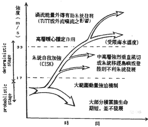
圖 20 影響颱風強度變化物理過程之理想示意圖。
