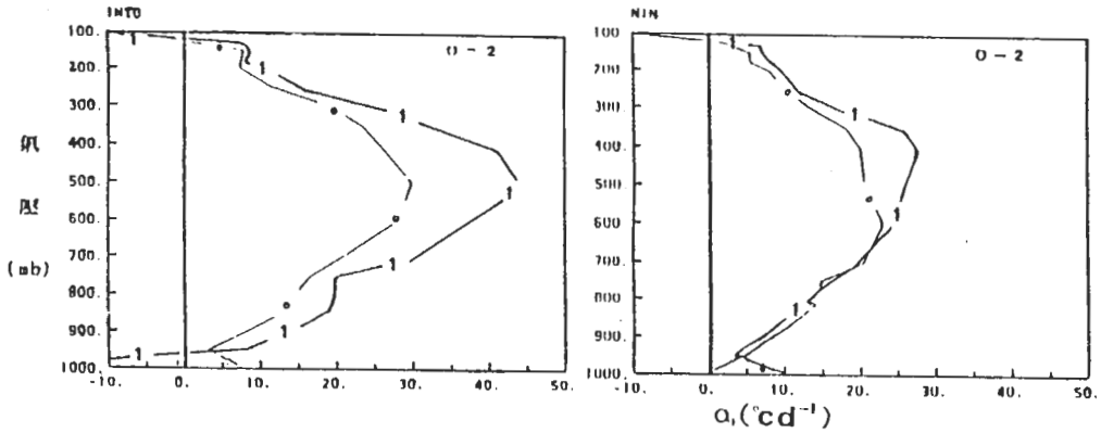
圖15 加強型(左)和非加強型(右)熱帶風暴(TS)於階段1(加強前)和0(加強前一天)之 0-2^{\circ} Q_1 垂直分佈圖。
