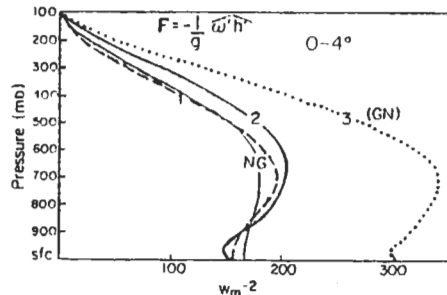
圖 9 0 \sim 4^\circ 之積雲垂直渦流能量傳送 ( F ) 垂直分佈圖。
