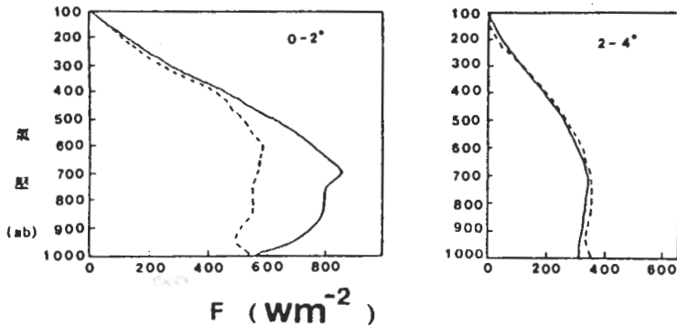
圖16 加強型和非加強型颱風於加強前(階段1)之 0-2^{\circ} 和 2-4^{\circ} 渦流能量垂直通量 ( F \equiv \omega' h' / g ) 垂直分佈圖。
