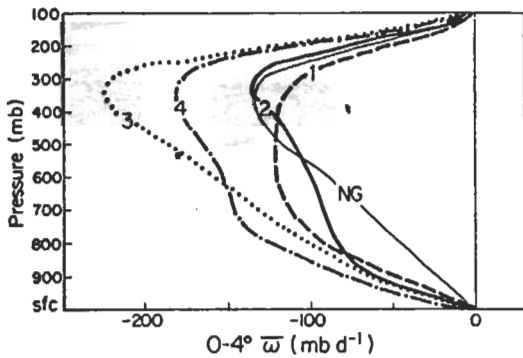
圖 7 發展個案合成 0 \sim 4^\circ 之平均垂直速度, 1, 2, 3, 4 表示不同階段, NG 為不發展個案之合成結果。
