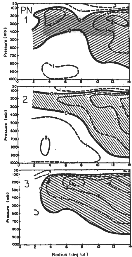
圖 5 不發展積雲簇 (NG) 於不同階段之切向風速徑向剖面分佈圖。
