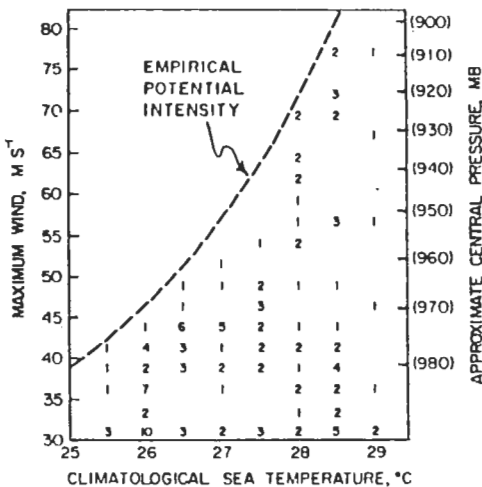
圖 17 北大西洋對應於某海水溫度，觀測達到某一最大強度之颱風個數。(摘自 Merrill, 1985 )
