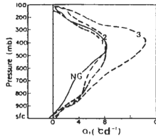
圖 8 0 \sim 4^\circ 之 Q_1 垂直分佈, 1, 2, 3, 為 GN 合成之三個階段, NG 為不發展個案 (NG 2) 合成結果。
