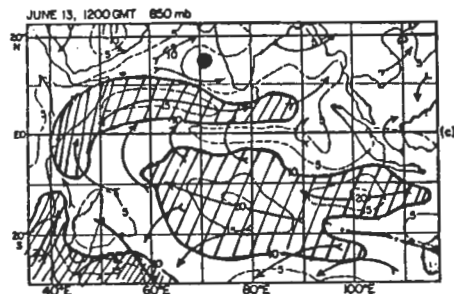
圖 13 北印度洋 TC 18-79 生成前之大範圍環流型式。TC 18-79 將在黑點處生成，斜線區表風速大於 10 kts。
