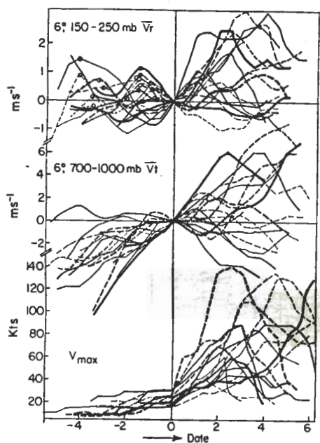
圖 12 1977 年 17 個颱風個案之強度，低層平均溫度和高層平均輻散場之時間變化。
