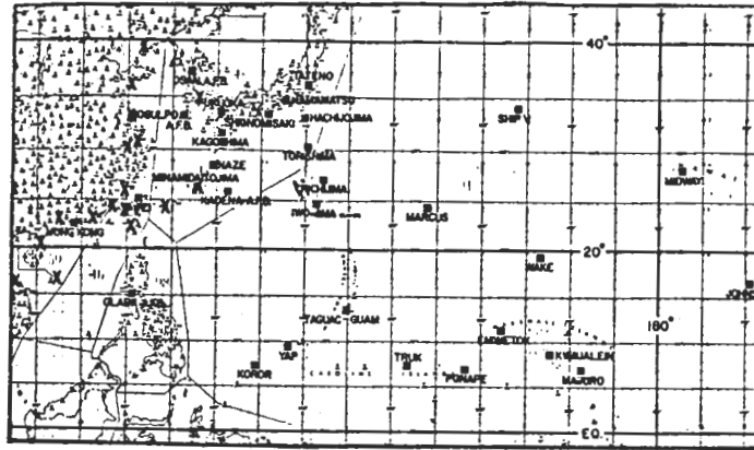
圖 3 西北太平洋地區颱風合成所採用之探空站分佈圖。
