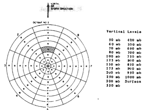
圖2 颱風合成座標,徑向可分8層,切向分8個方位。垂直方向解析度為23層,方位1表示北方。
