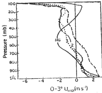
圖 6 不發展 (NG) 和發展 (GN) 合成 (1, 2, 3 表不同階段) 之 0 \sim 3^\circ 東西向風速垂直分佈圖。
