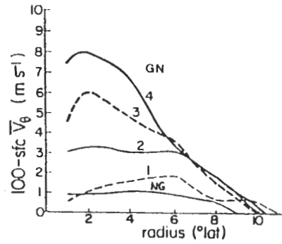
圖11 對流層平均之切向風速徑向分佈圖。
