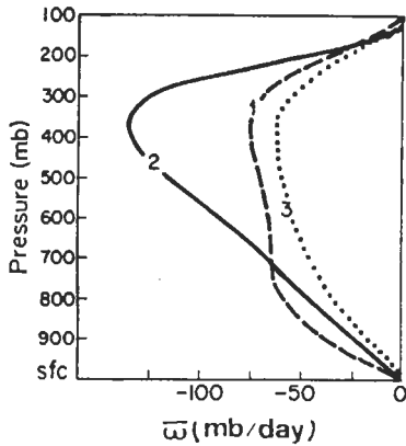
圖 4 不發展之積雲簇 (NG) 於不同階段之 0 ~ 4° 垂直運動。
