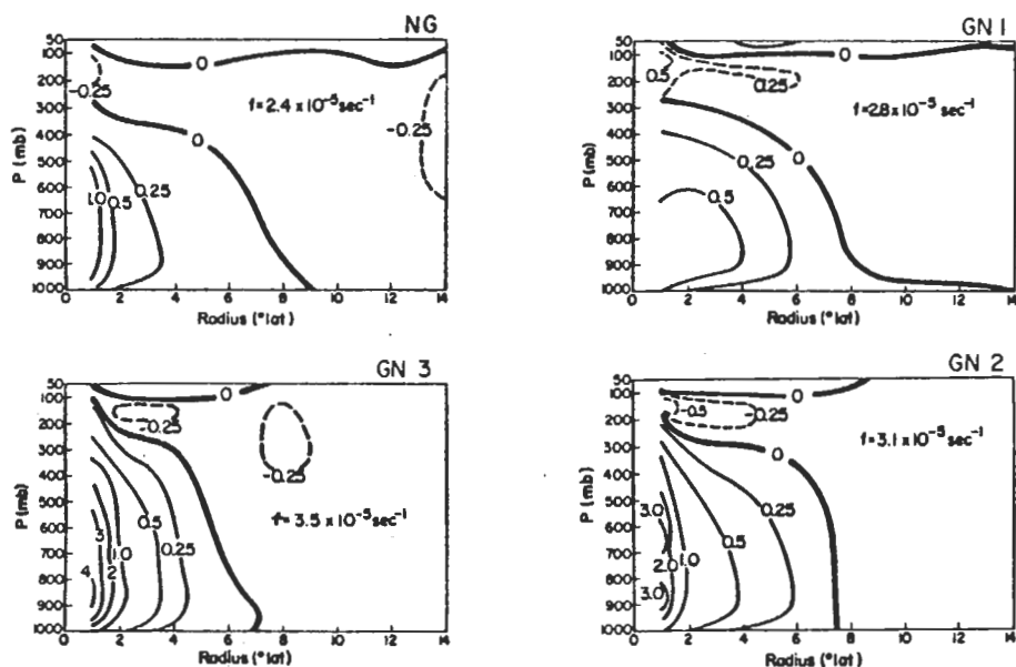
圖 10 相對渦度 (以 f 表示) 之徑向剖面圖。
