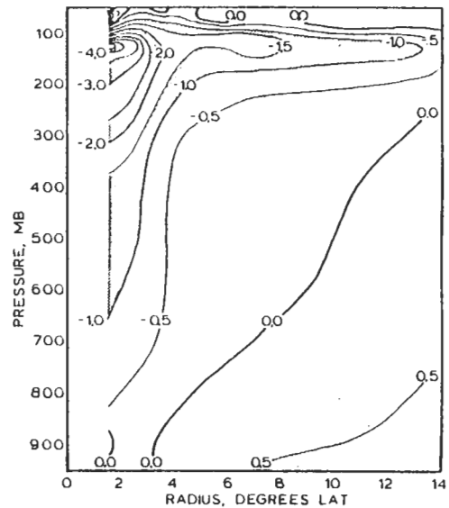
圖 18 加強中颱風和不加強中颱風 ( 強度 \geq 64 kts ) 合成溫度之差值。
