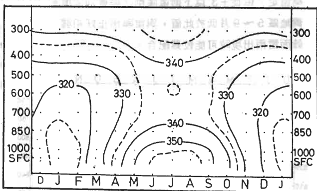
圖 16: 台灣地區逐月相當位溫分布圖。(單位 ^\circ\text{K} )
