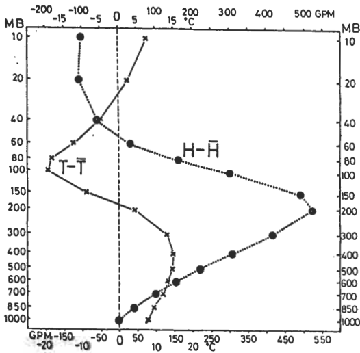
圖 20: 台灣區年平均大氣曲線之高度(H)及溫度(T)與標準大氣曲線之高度(H̄)和溫度(T̄)之偏差變化圖。
