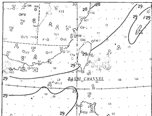
圖十一 民國七十年八月台灣近海海水面月平均溫度分佈圖(單位 ^{\circ}\text{C} )。
