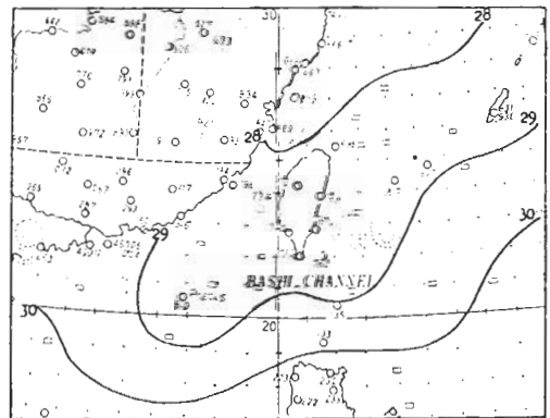
圖十 民國七十年七月台灣近海海水面月平均溫度分佈圖(單位 ^{\circ}\text{C} )。
