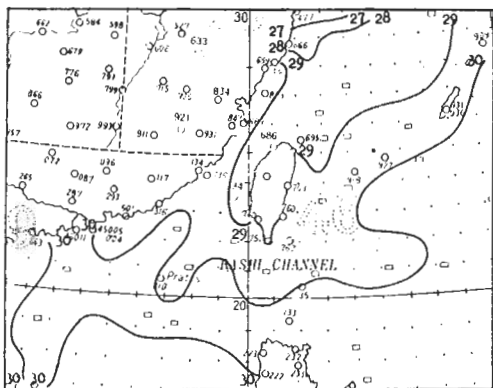
圖十二 民國七十年九月台灣近海海水面月平均溫度分佈圖(單位 ^{\circ}\text{C} )。
