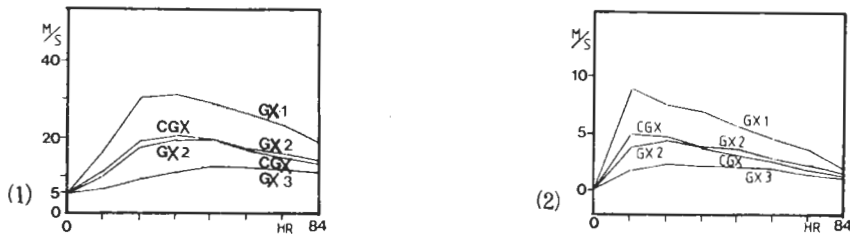
圖 11：第二部分實驗中，各個個案的水平風場最大值隨時間的變化
