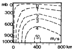
圖 3：初始切綫風場剖面圖
