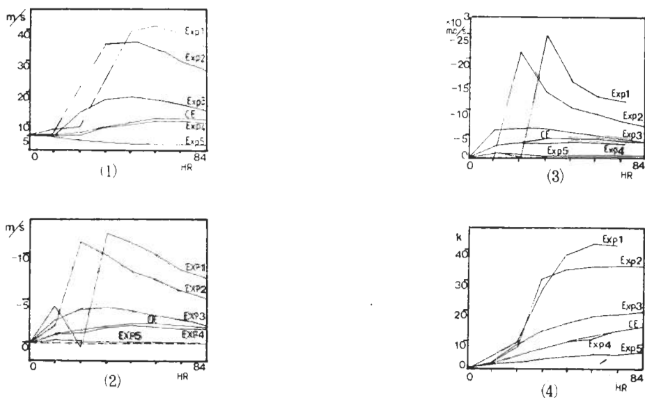
圖 4 : 第一部分實驗中各個個素的四個物理量最大值隨時間的變化情形 (1) 900 MB 切線風速 (2) 900 MB 徑向風速 (3) 450 MB 垂直風速 (4) 450 MB 位溫變差 ( \theta - 329.48^\circ\text{K} )
